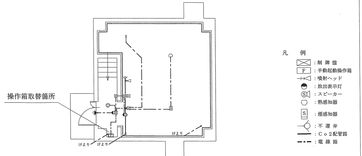
#16通信局舎(2F)平面図 S=1:100
