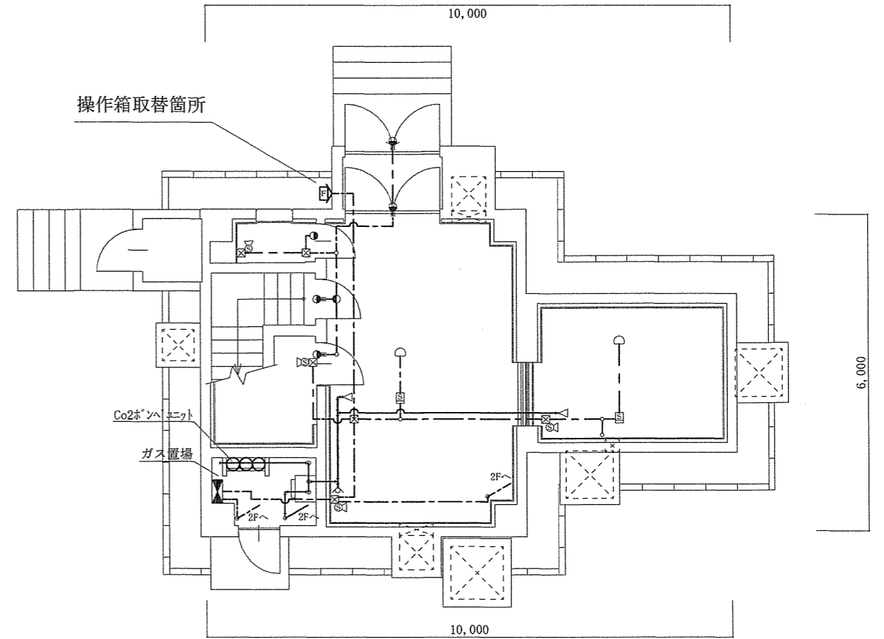
#16通信局舎(1F)平面図 S=1:100
