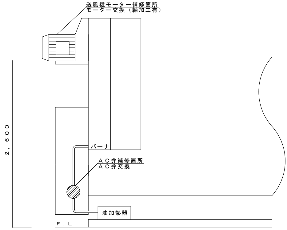
2号ボイラー側面図 S = 1 : 25
