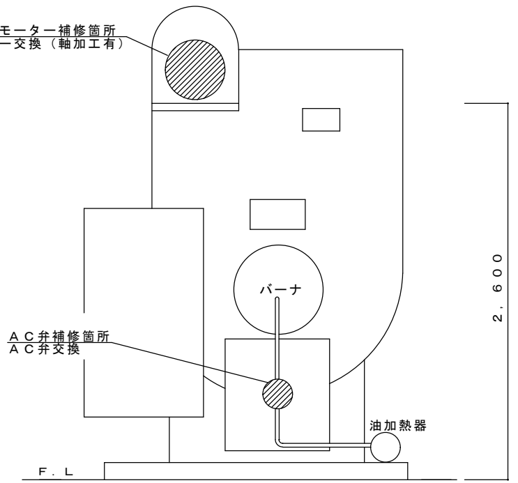
1号ボイラー立面図 S = 1 : 25
