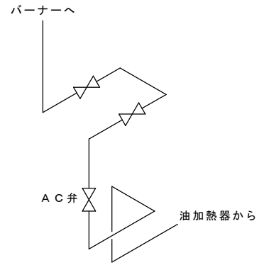
A C 弁接続系統図 S = 1 : 10
