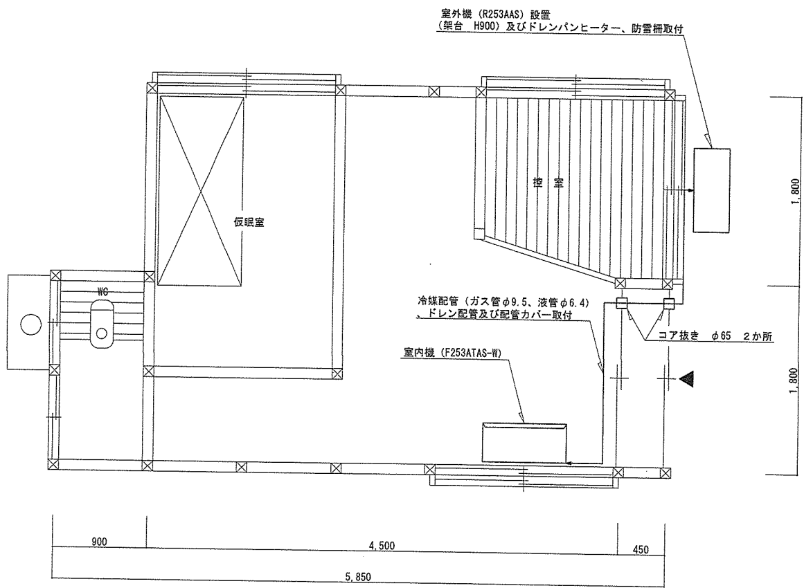
# 2 6 警衛所分哨所 平面図 縮尺 1 : 50
