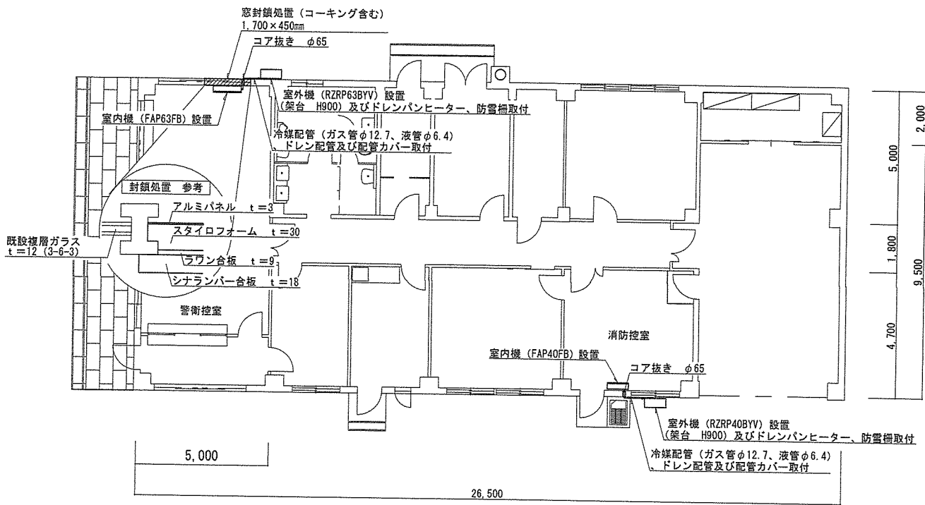
# 1 3 警衛所平面図 縮尺 1 : 200
