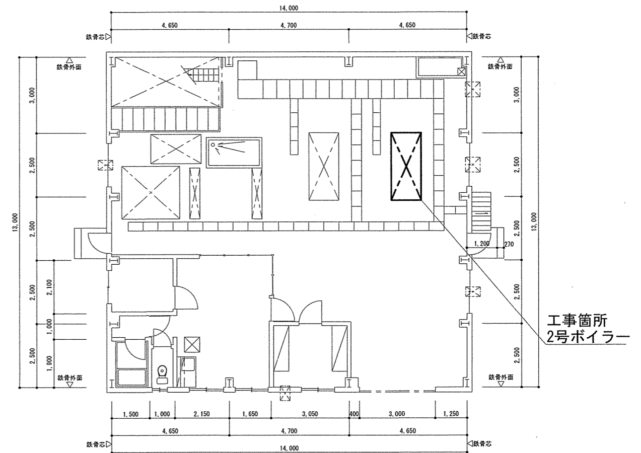
#6ボイラー室平面図 S = 1/150
