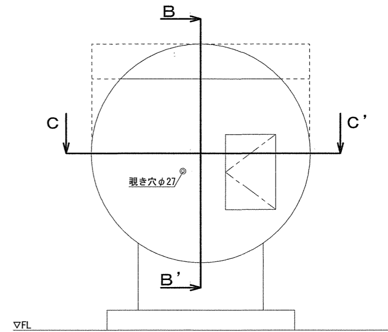
2号ボイラー後方立面図 S=1:30
