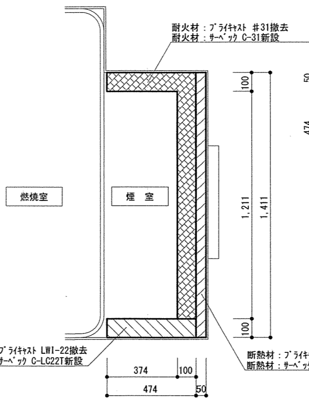
B-B' 断面図 S=1:20
