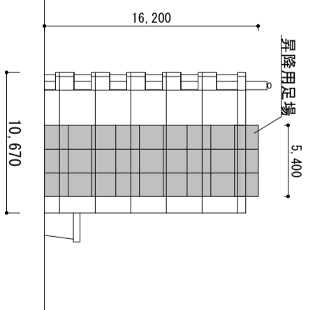
北東側立面図 S=1: 400
