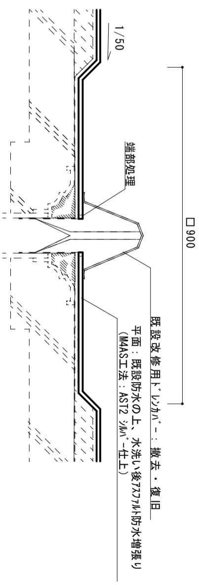
ルーフトップ断面詳細図 S=1:10
