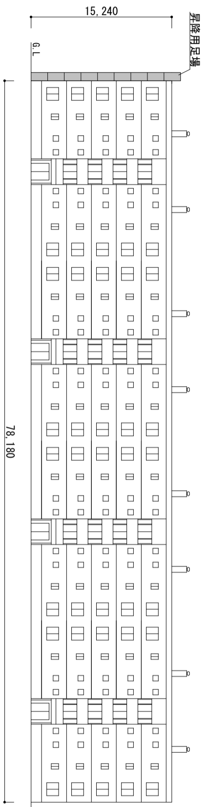
南東側立面図 S=1: 400
