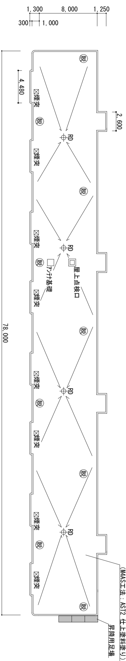
屋根伏図 S=1: 300
