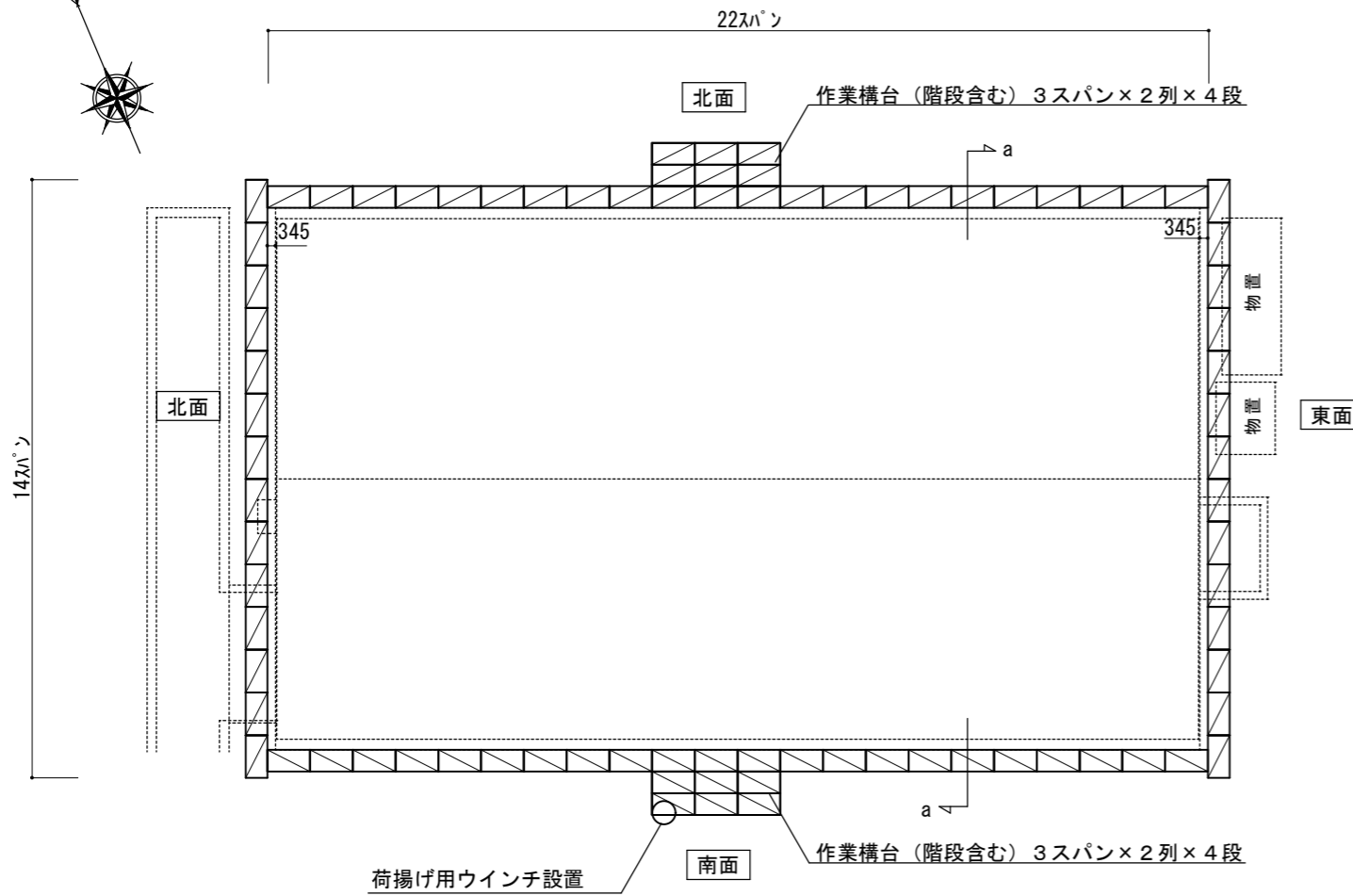
#20 体育館 屋根伏図
