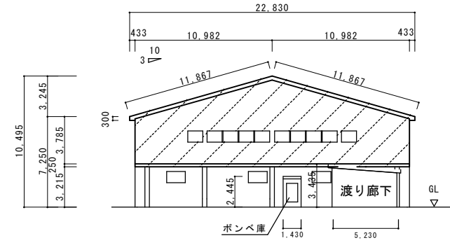
#20 体育館 西面立面図
