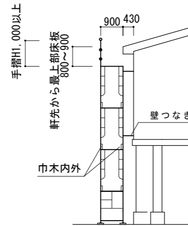
a断面図 S=1/150
