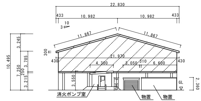
#20 体育館 東面立面図
