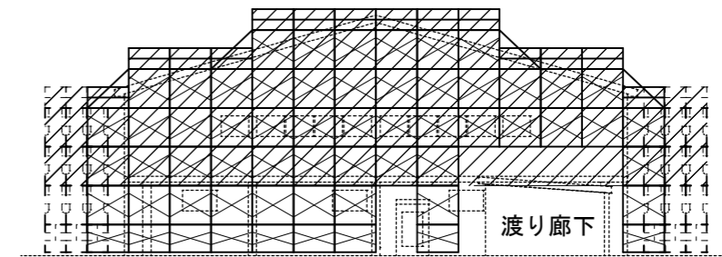
#20 体育館 西面立面図
