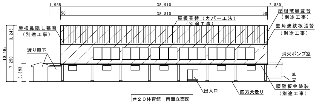
#20 体育館 南面立面図
