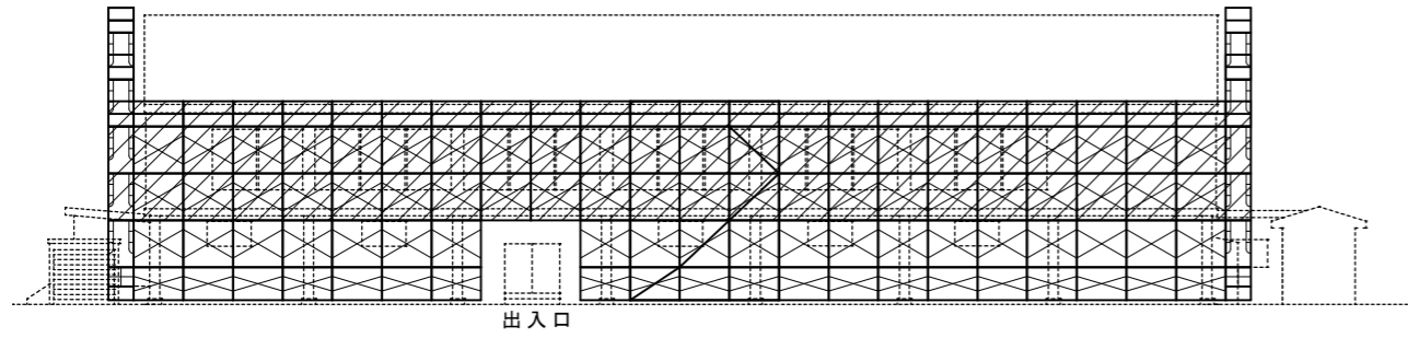
#20 体育館 北面立面図
