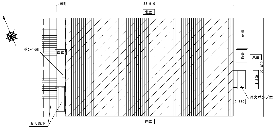
#20 体育館 屋根伏図
