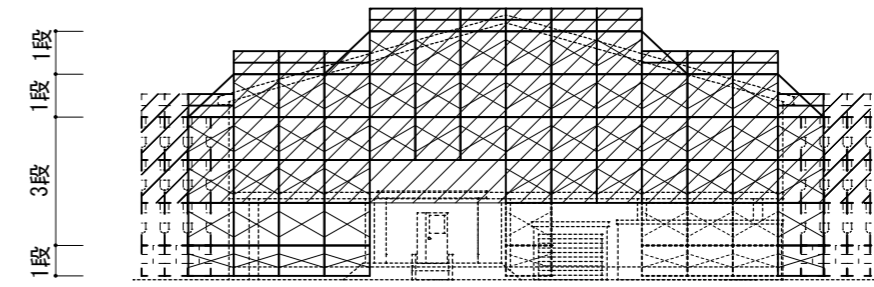
#20 体育館 東面立面図
