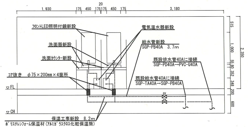
新設立面図 S=1/50
