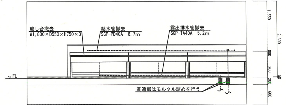
撤去立面図 S=1/50
