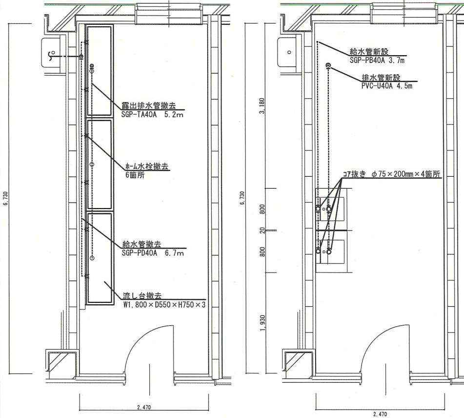
撤去平面図 S=1/50
