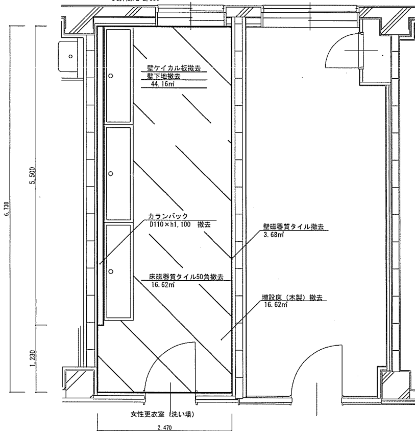
撤去図1/50
