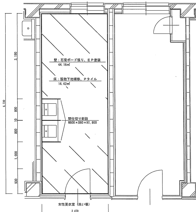
改修図1/50
