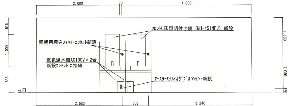
詳細図 S=1/50
