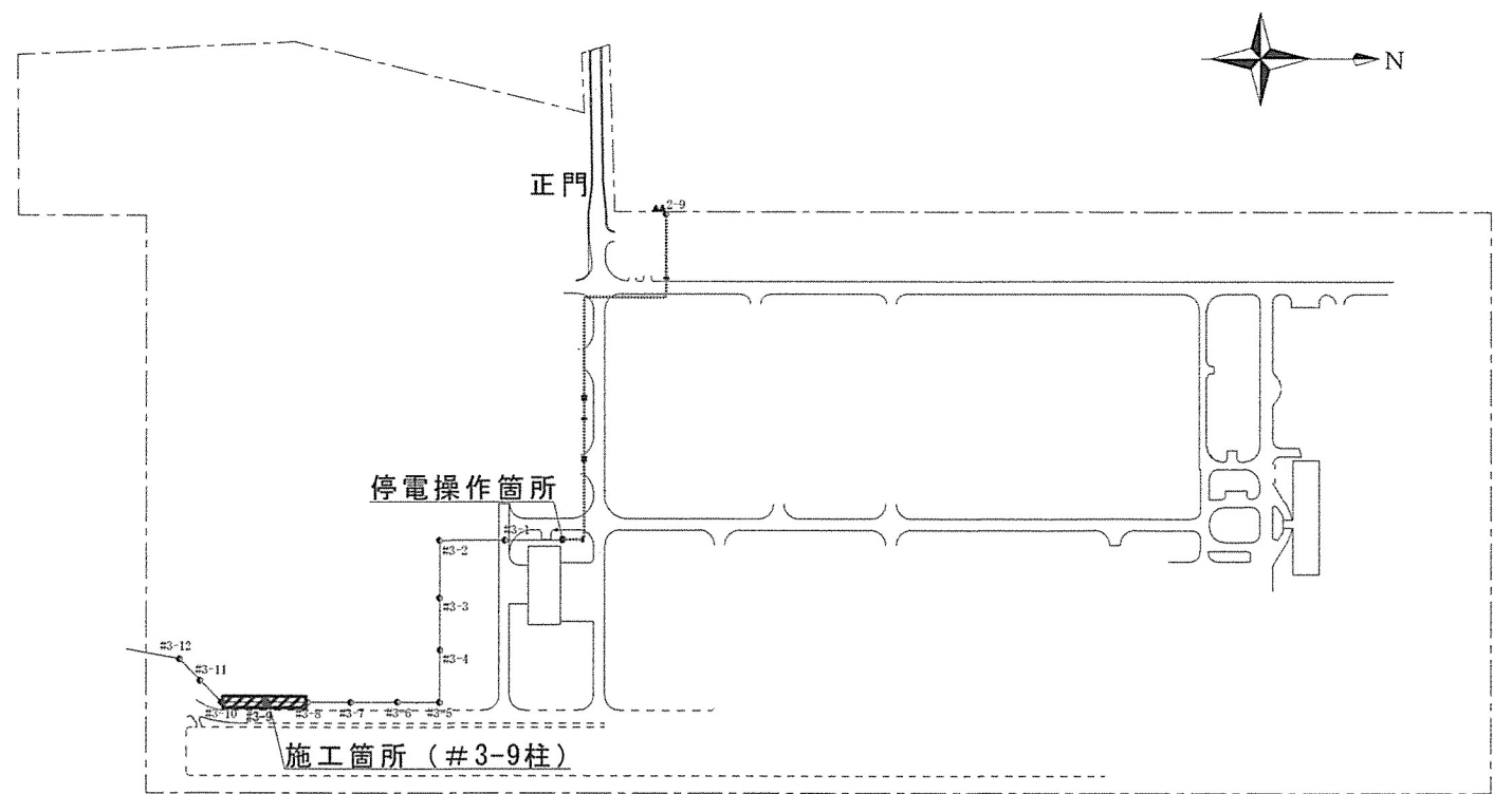
駐屯地構内外線図 S=1/5,000
