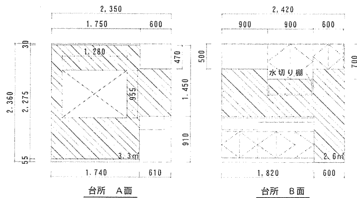
展開図 S=1/50
