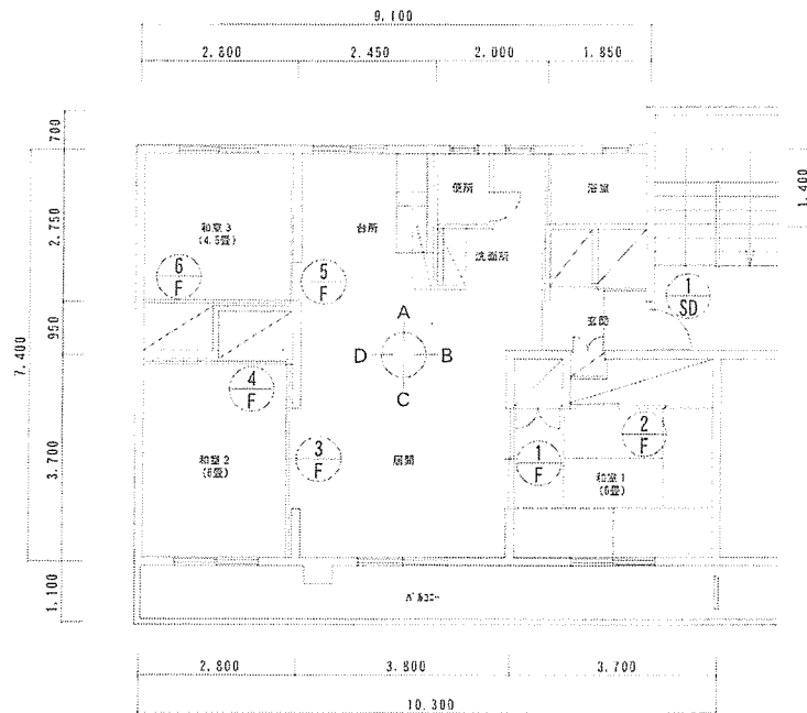
各戸平面図 S=1/100
