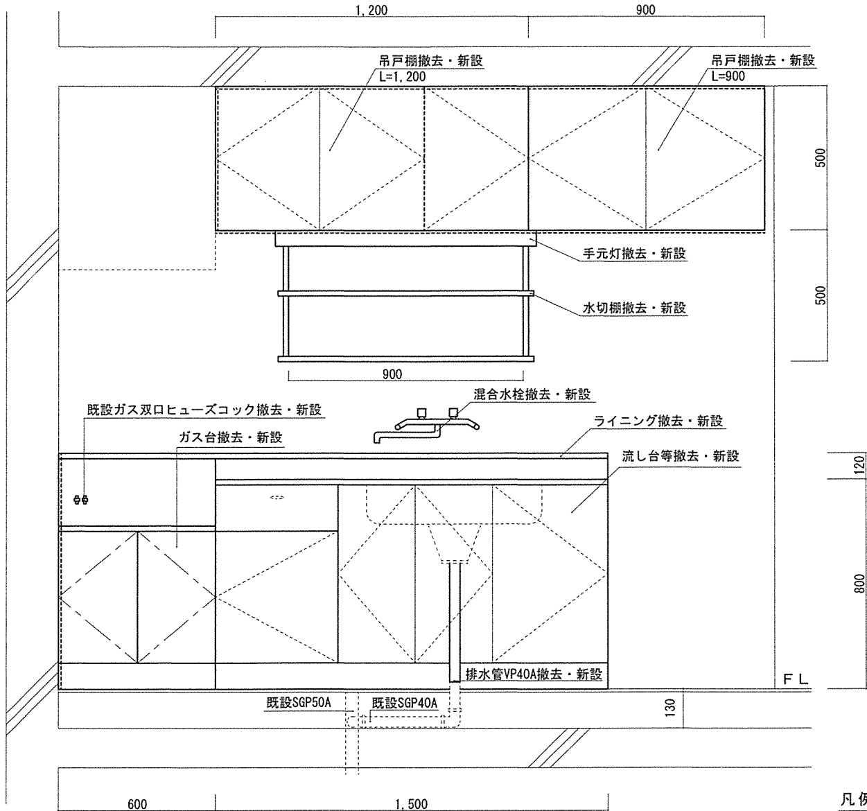
既設台所 標準断面図 (A面) S=1/20
