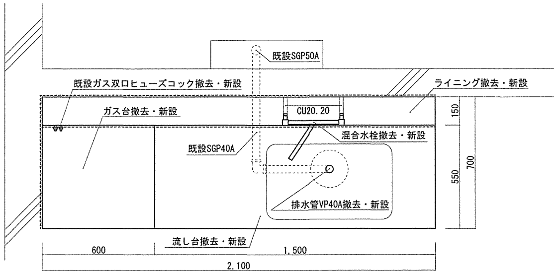
既設台所 標準平面図 S=1/20
