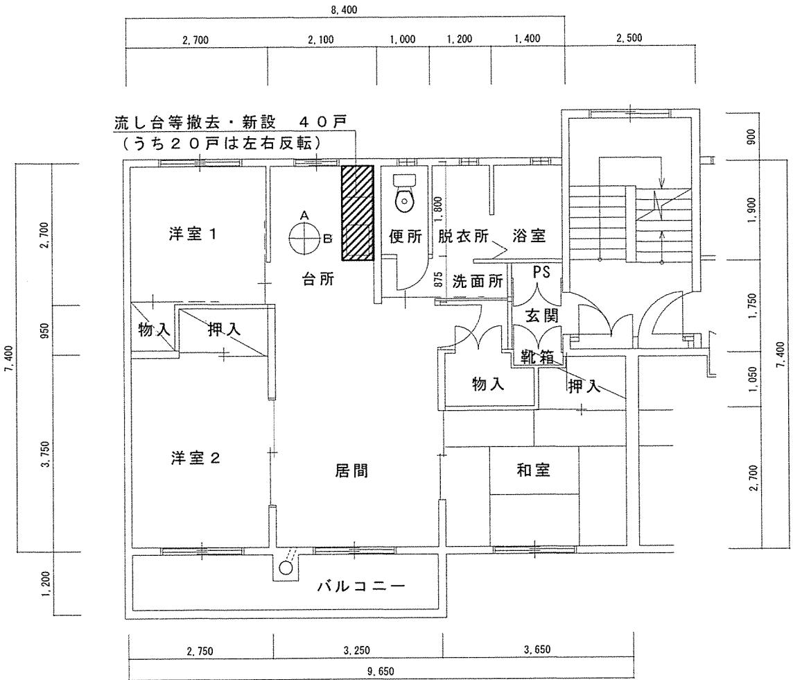
東宿舍4号棟・8号棟（共通） 平面図 S=1/100
