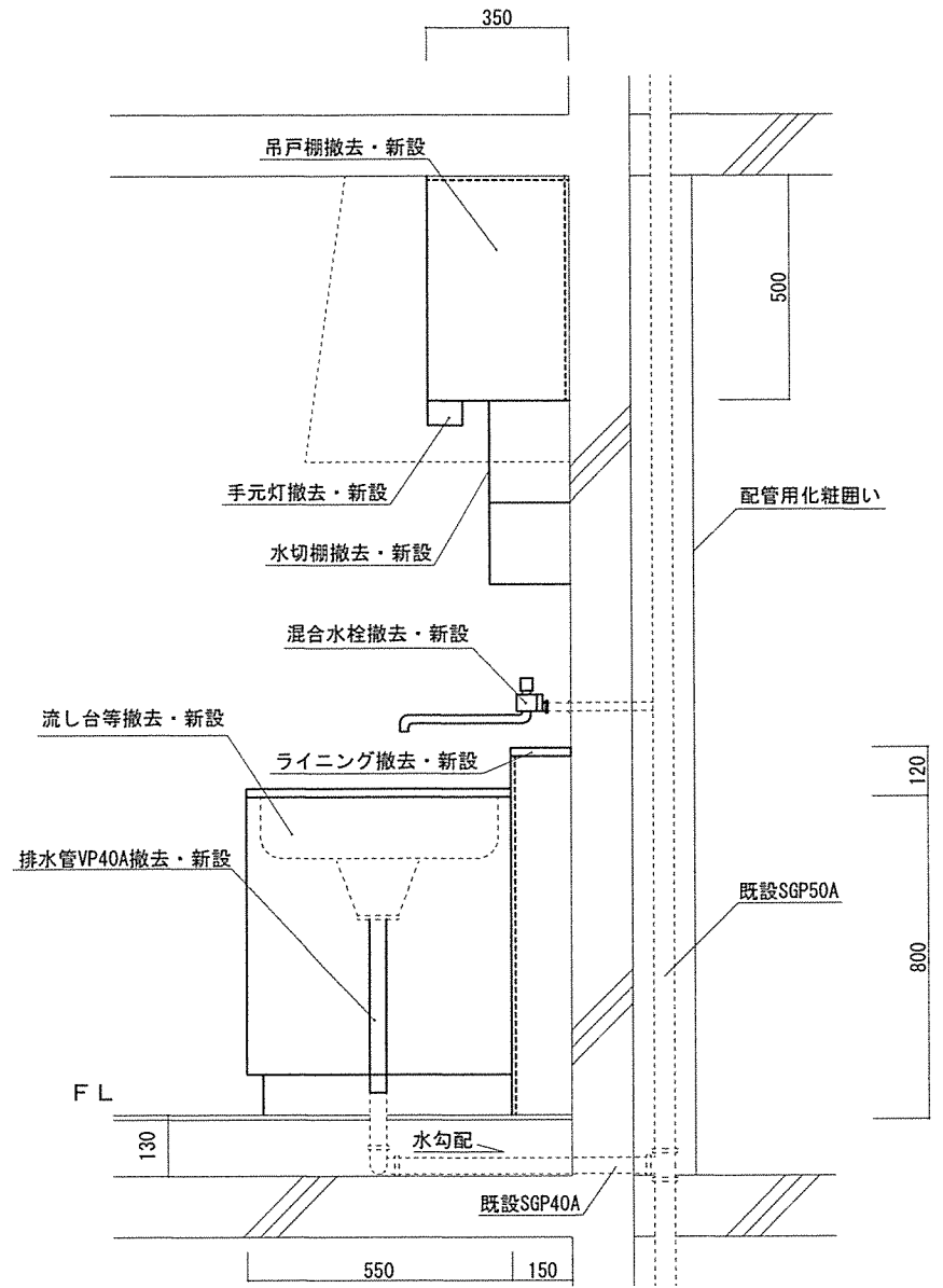
既設台所 標準断面図 (B面) S=1/20
