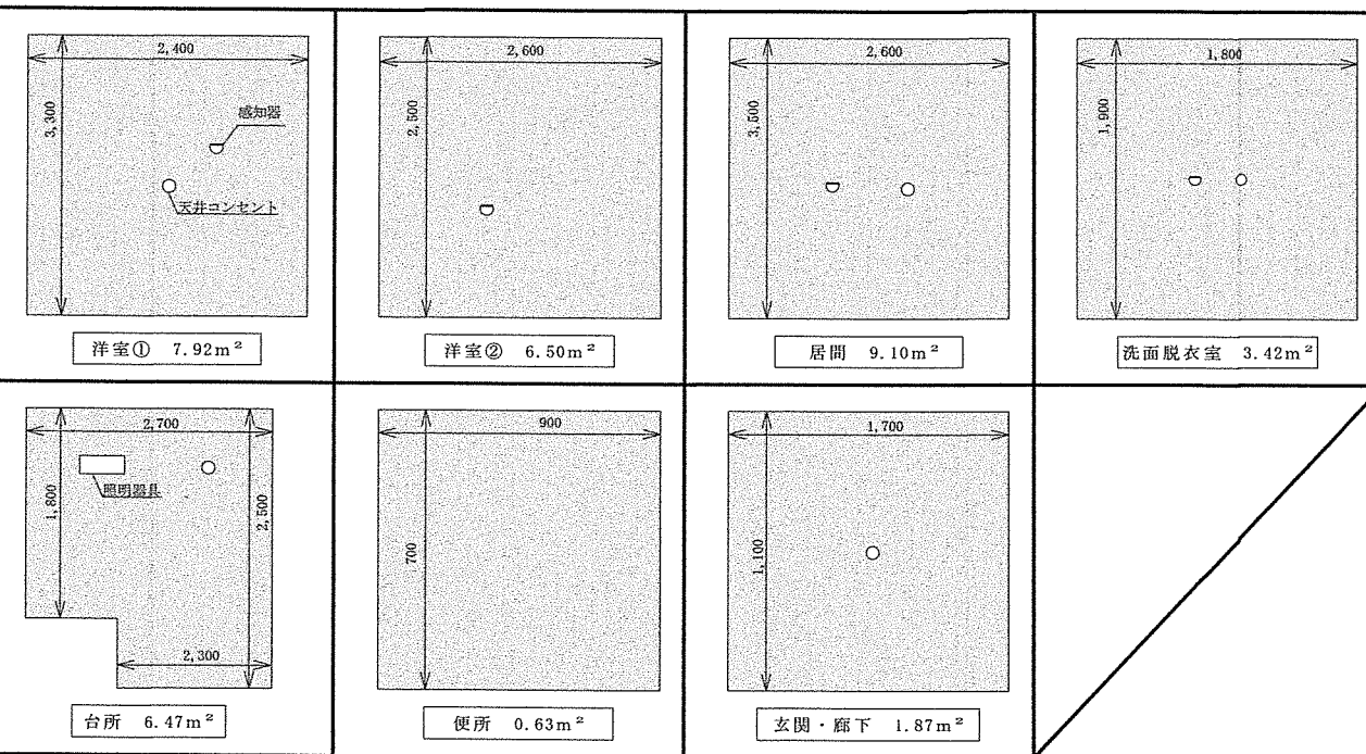
幌別宿舍天井伏図 S=1:X
