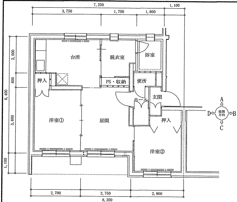
幌別宿舍平面図 S=1:90
