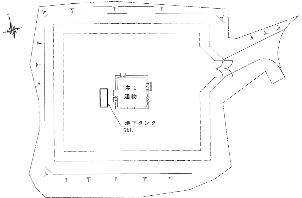
配置図 NO SCALE
