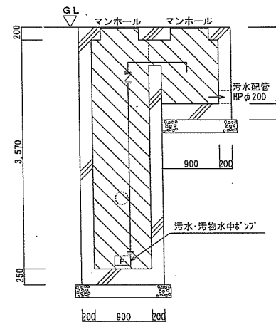
A-A'断面図 S=1/60
