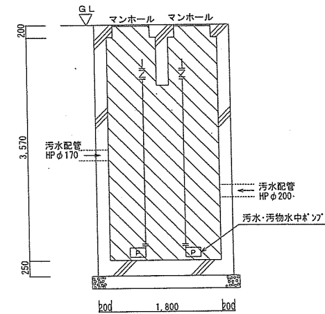
B-B'断面図 S=1/60
