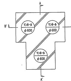
平面図 S=1/60
