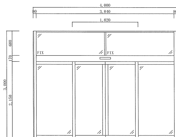
自動ドア建具表 S=1:60
