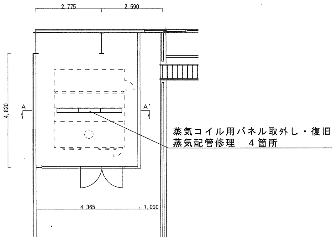
体育館（2階）機械室平面図 S=1:100
