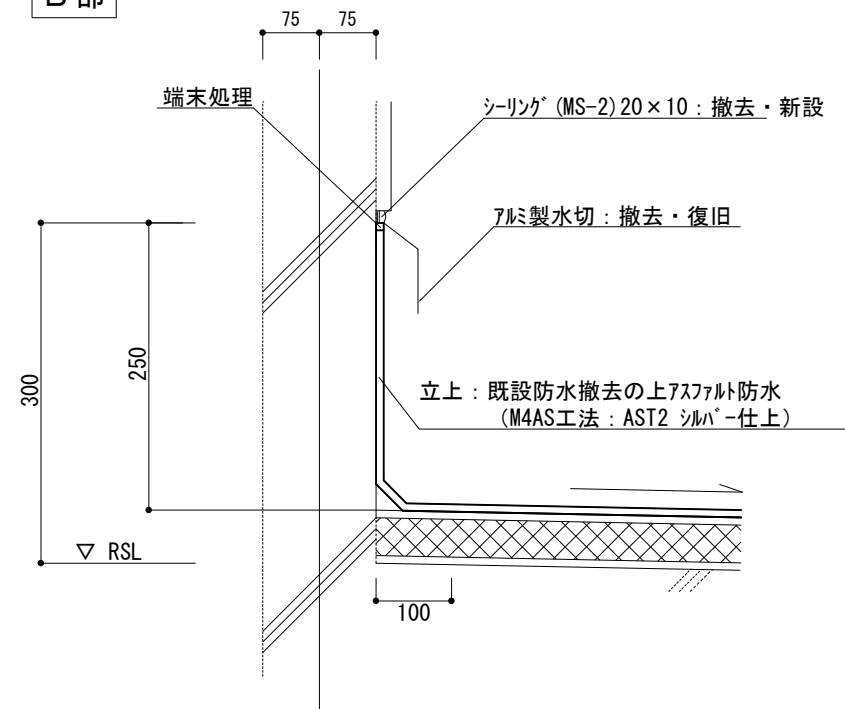
#3306水切部断面詳細図 S=1:10
