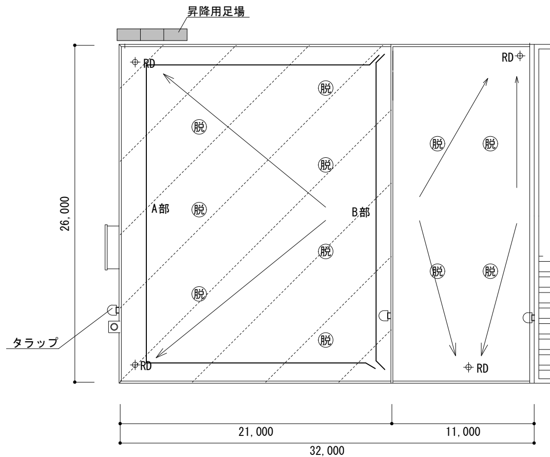
#3306屋根伏図 S=1 : 300
