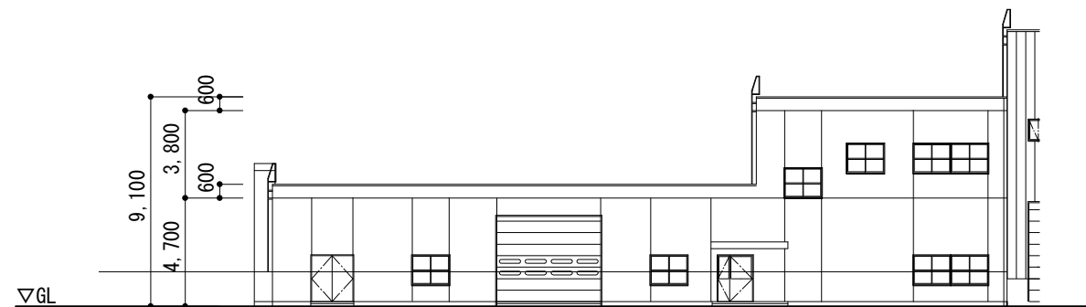
#3306南側立面図 S=1 : 300
