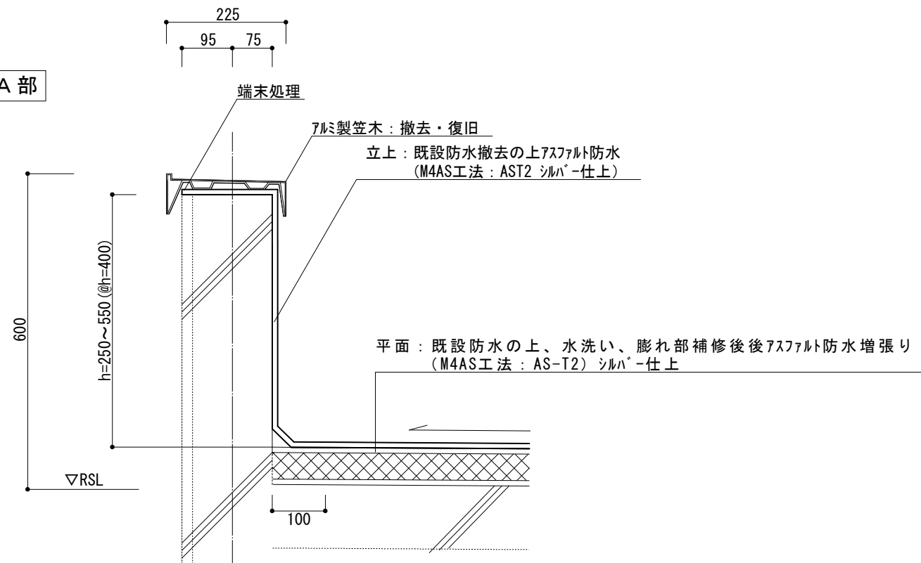
#3306パラペット断面詳細図 S=1:10
