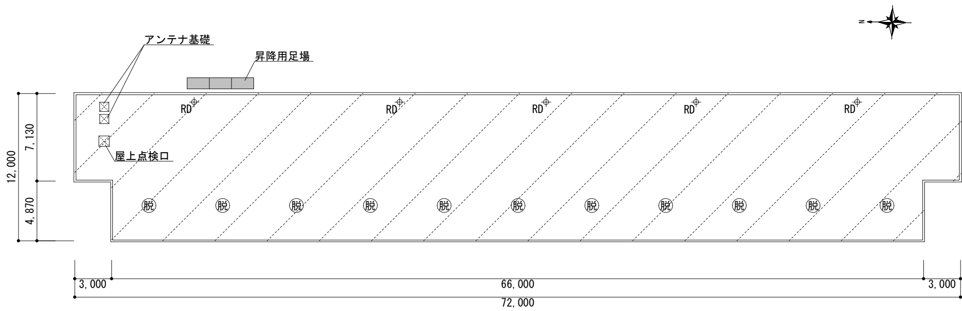
#3112屋上平面図 S=1 : 300
