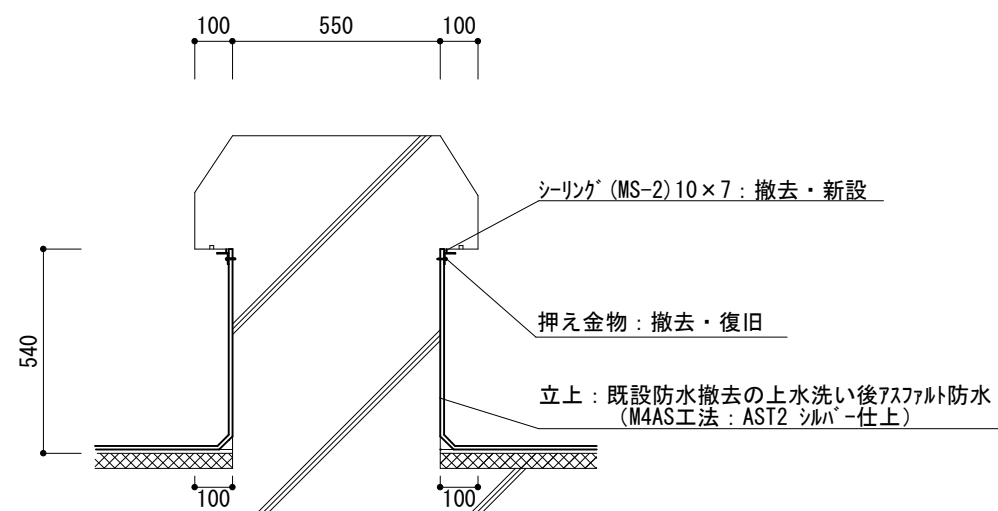
#3112 アンテナ基礎詳細図 S=1:20
