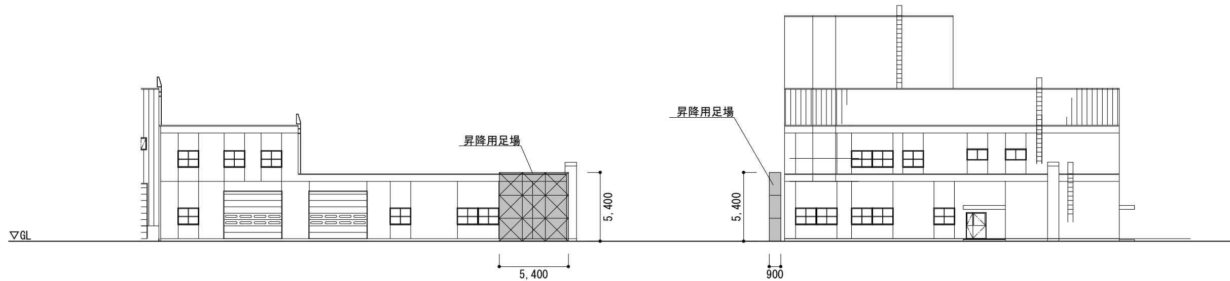
#3306北側立面図 S=1 : 300
