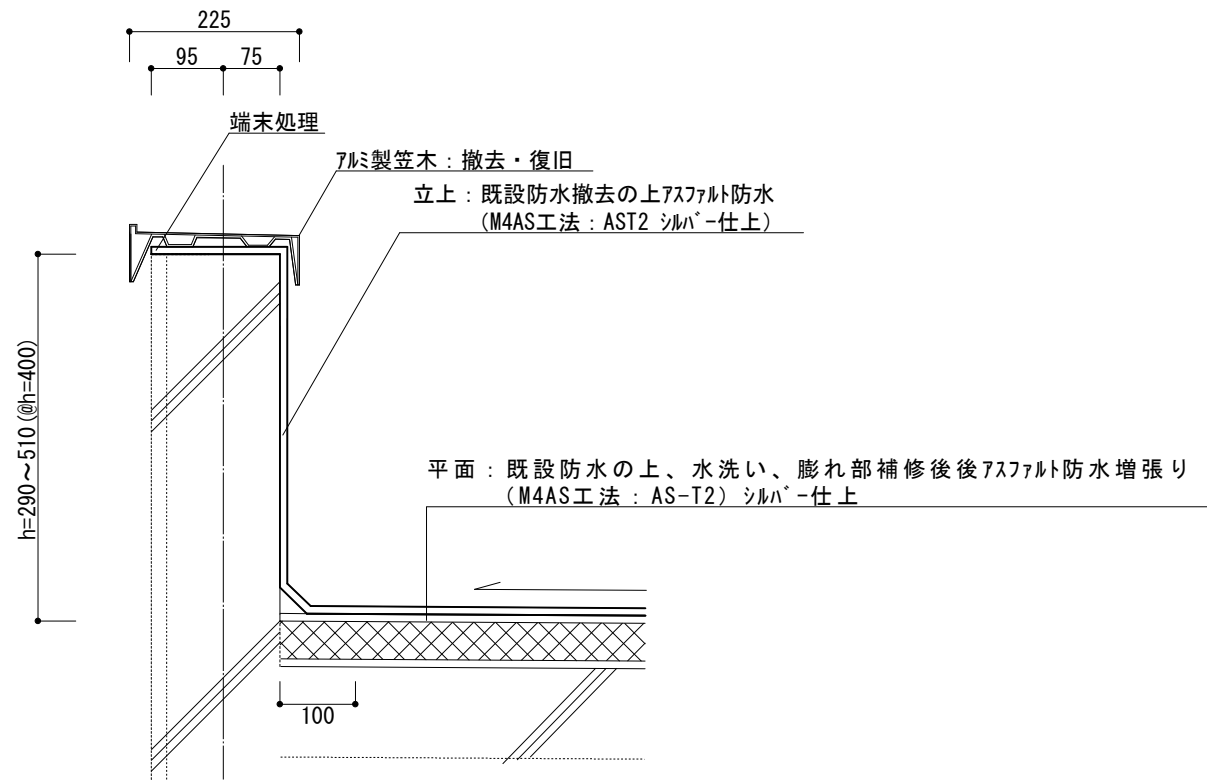
#3112パラペット断面詳細図 S=1:10
