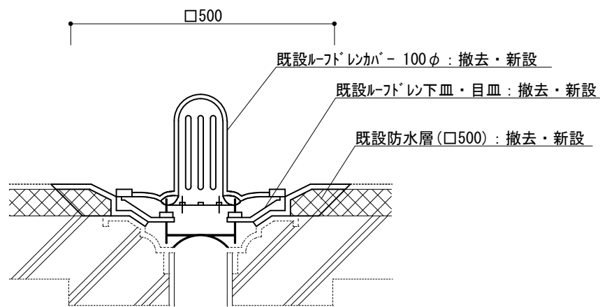
#3306ルーフトレン断面詳細図 S=1:10
