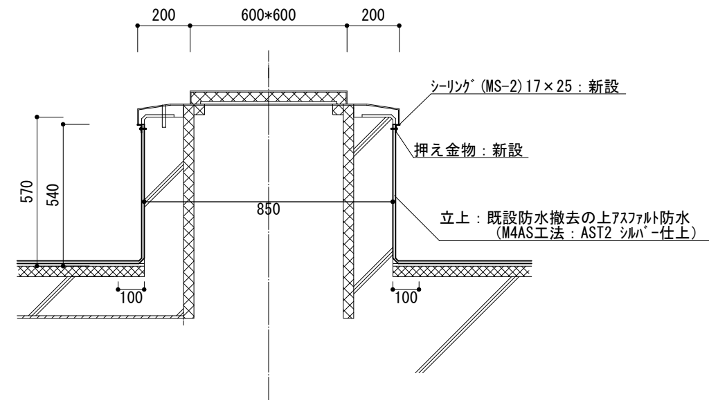
#3112屋上点検口詳細図 S=1:20
