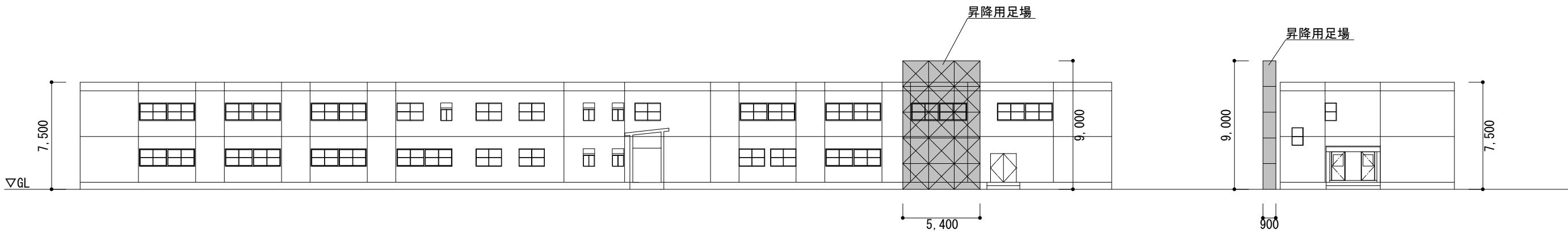
#3112西側立面図 S=1 : 300
