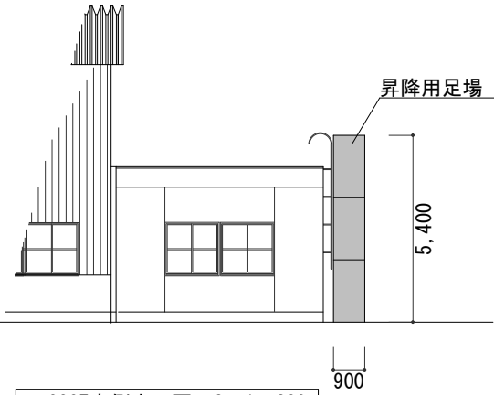
#2327東側立面図 S=1 : 300
