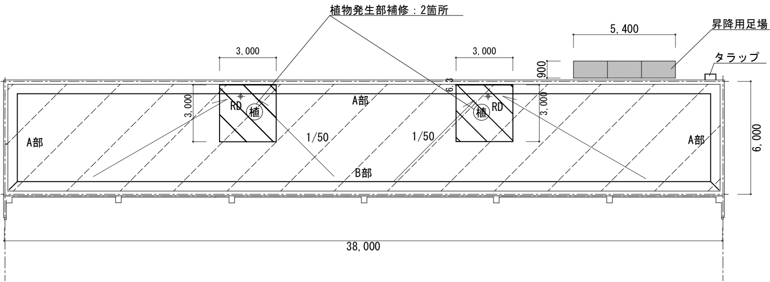
#2327屋上平面図 S=1 : 200
