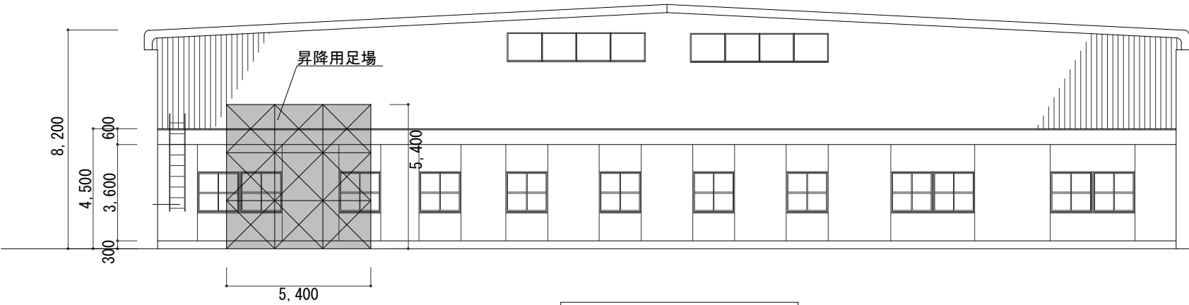
#2327北側立面図 S=1 : 200
