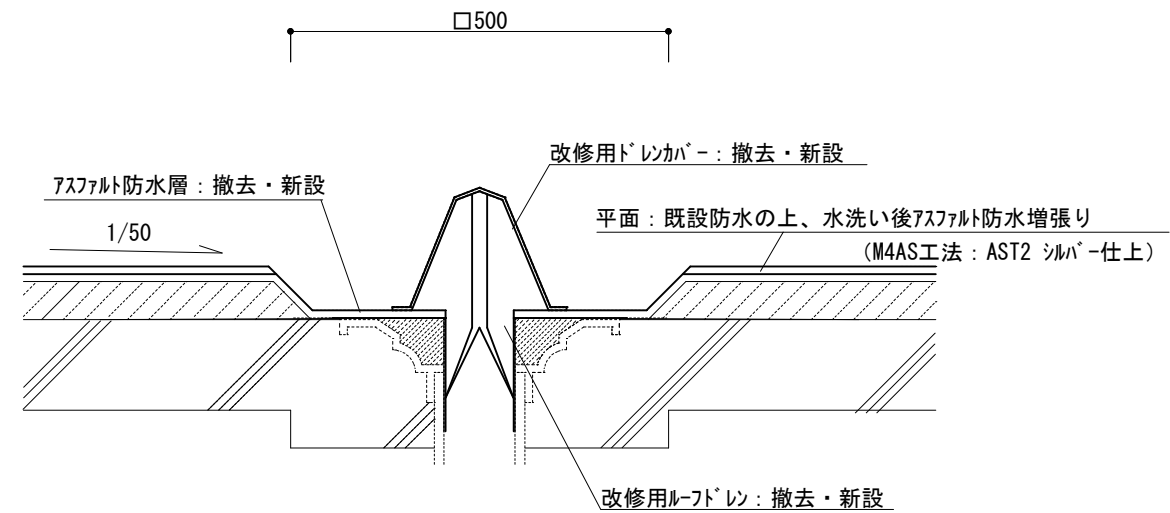
#2310ルーフトレン断面詳細図 S=1:10
