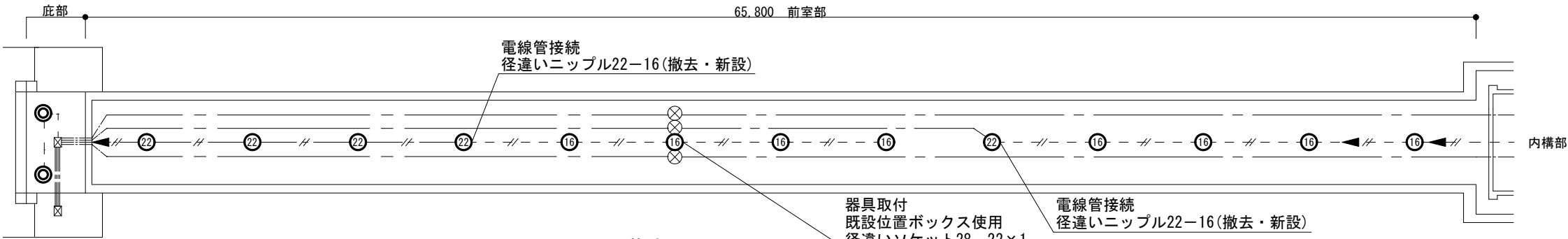
# 3 2 弾薬庫照明器具平面図
