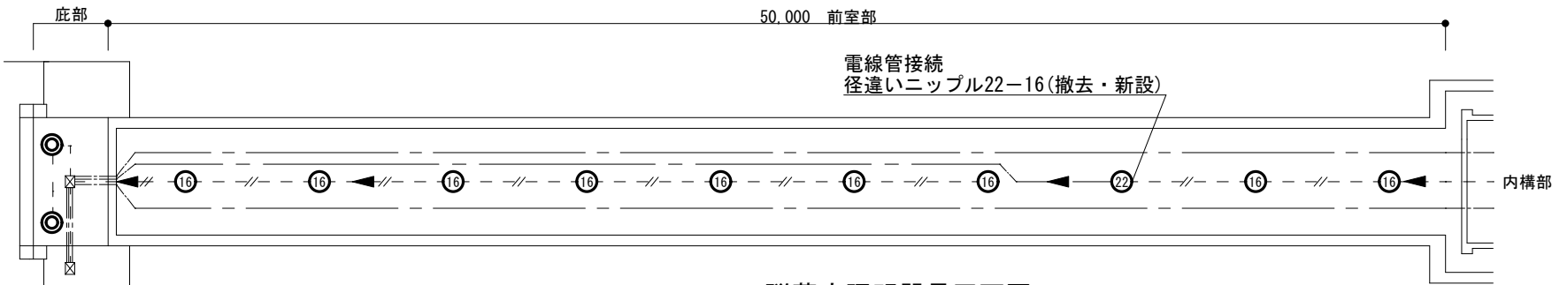
# 2 3 弾薬庫照明器具平面図
