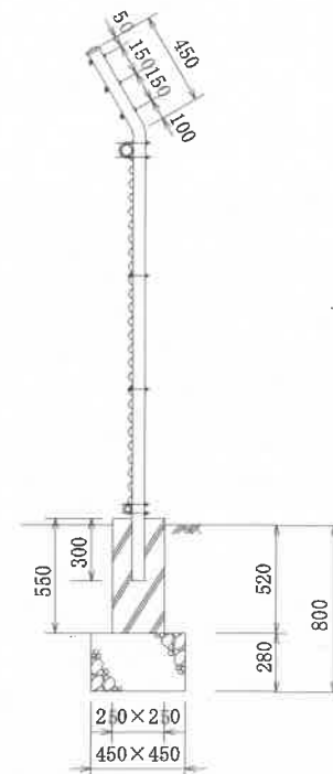
側面図 S=1:40
