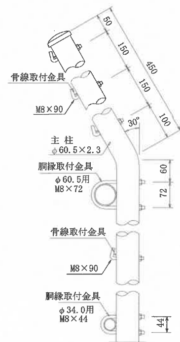
主柱・胴縁・骨線取付部詳細図 S=1:10
