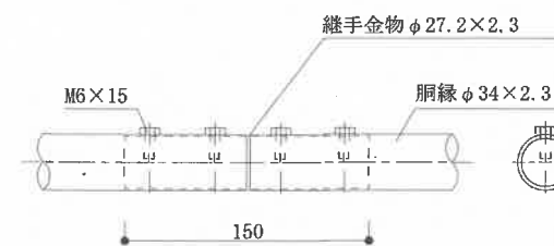
(新設) 胴縁継手部標準図 S=1:5
