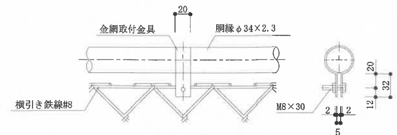
(新設) 金網取付金具標準図 S=1:5
