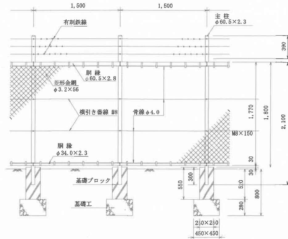
正面図 S=1:40
