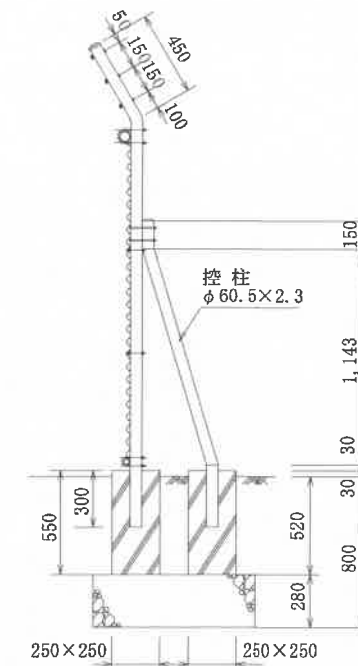
側面図 S=1:40
