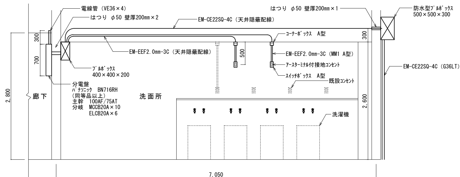
洗面所（A面）配線・機器取付詳細図 S=1:50
