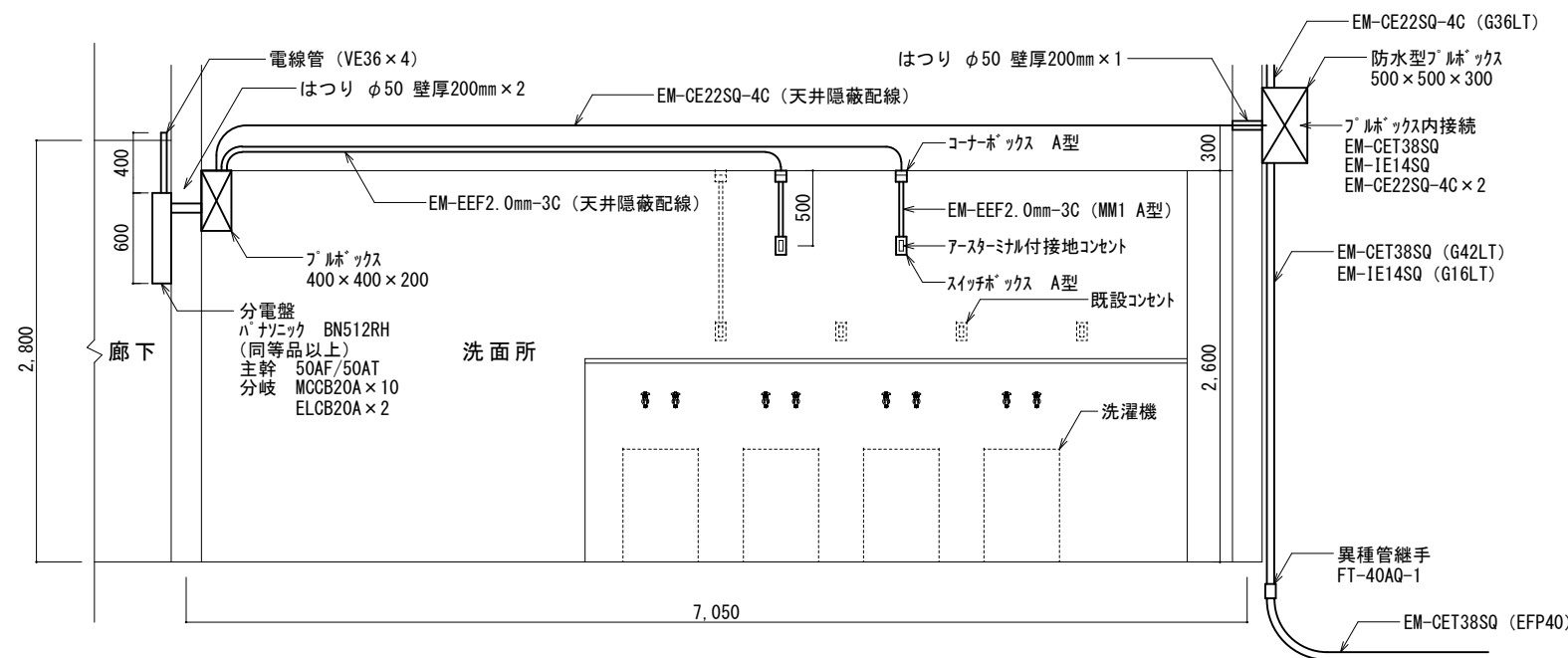
洗面所（A面）配線・機器取付詳細図 S=1:50
