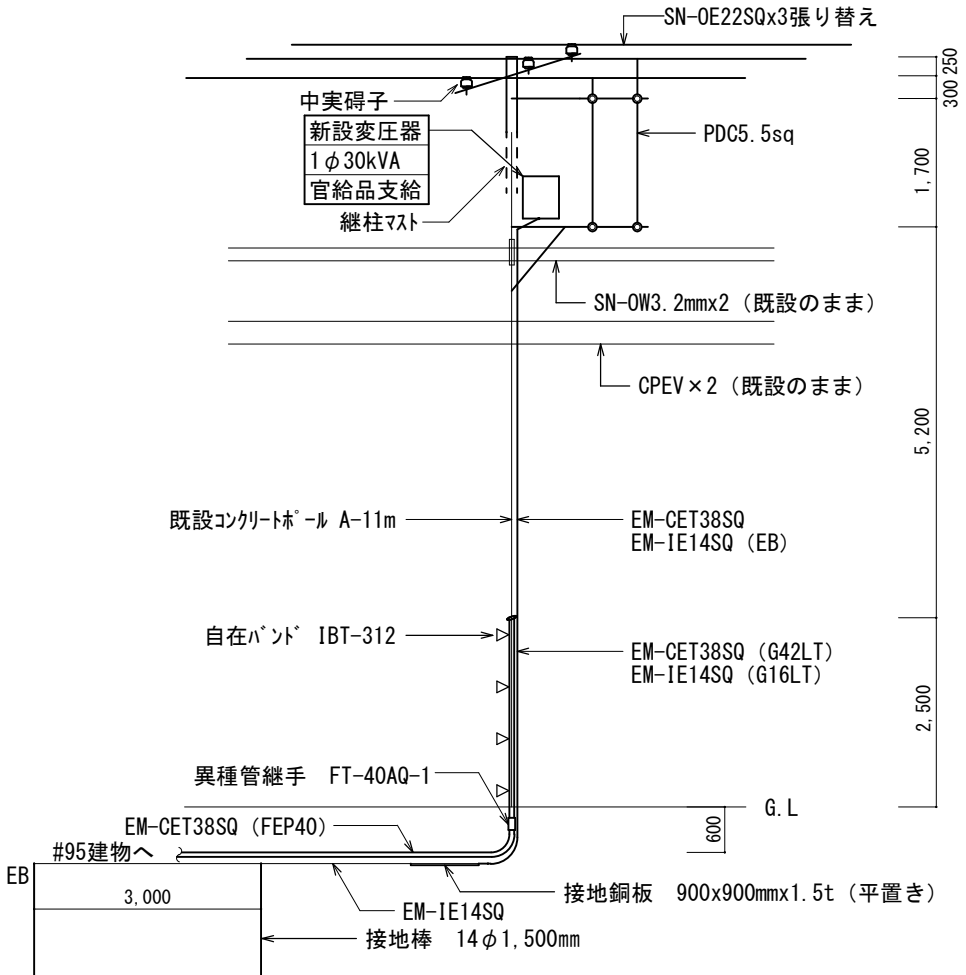
幹6-6号柱改修後装柱図 S=1:100
