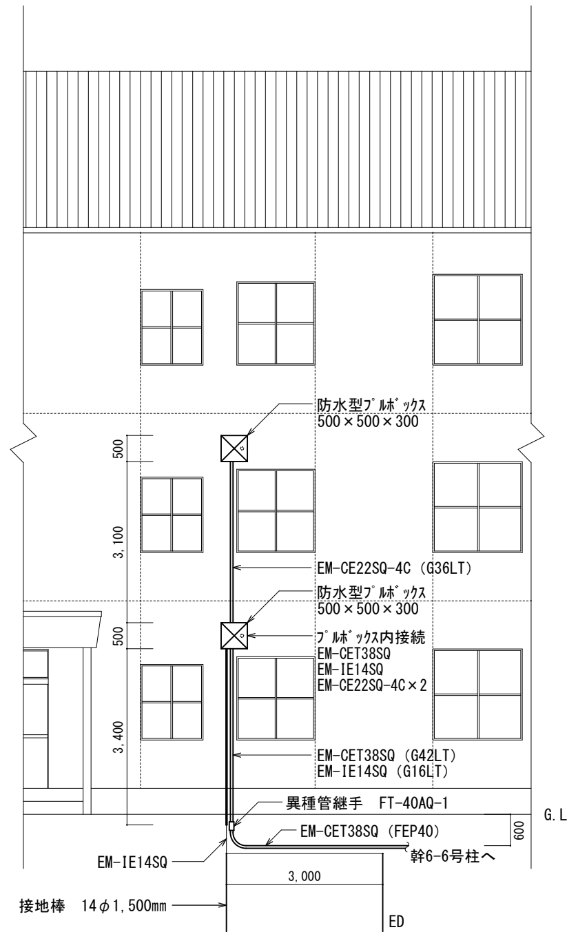
#95建物屋外配管立面図 S=1:100
