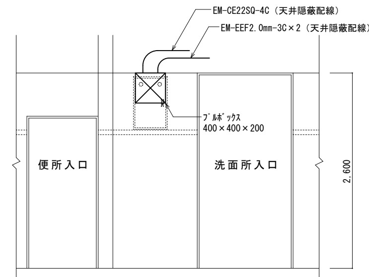
洗面所（B面）配線・機器取付詳細図 S=1:50
