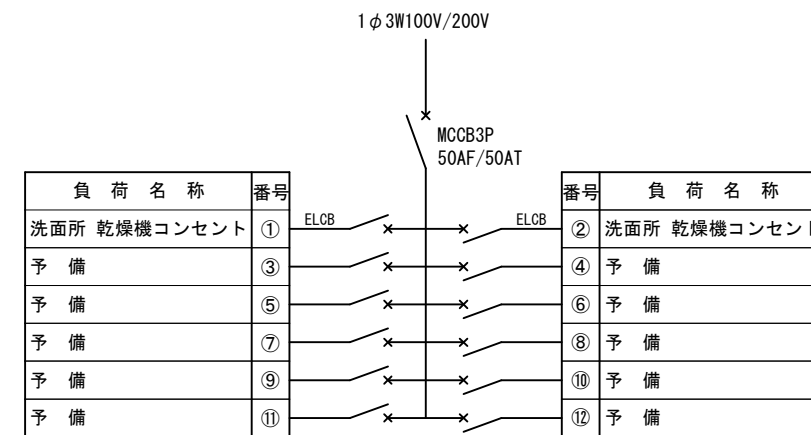
分電盤回路図 NO SCALE
