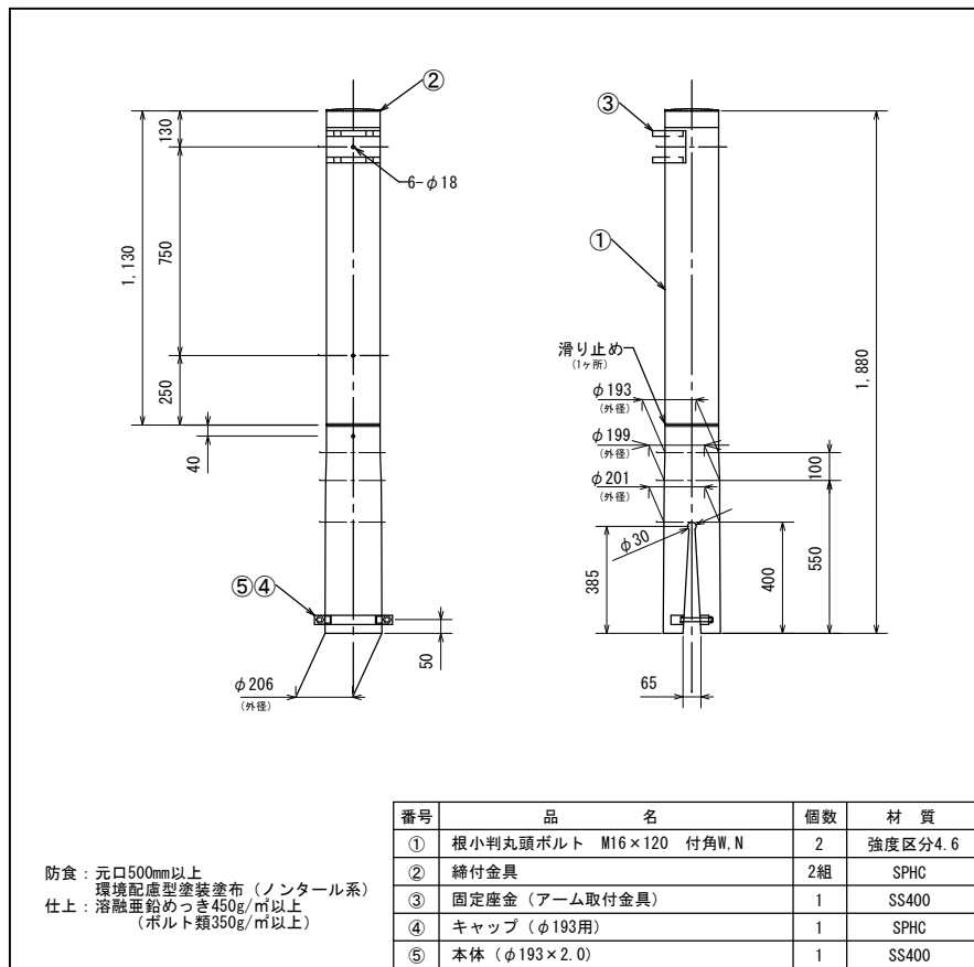
継柱ﾏｽﾄ仕様図 NO SCALE
