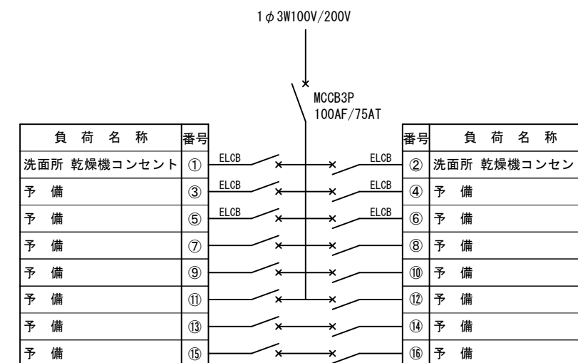
分電盤回路図 NO SCALE
