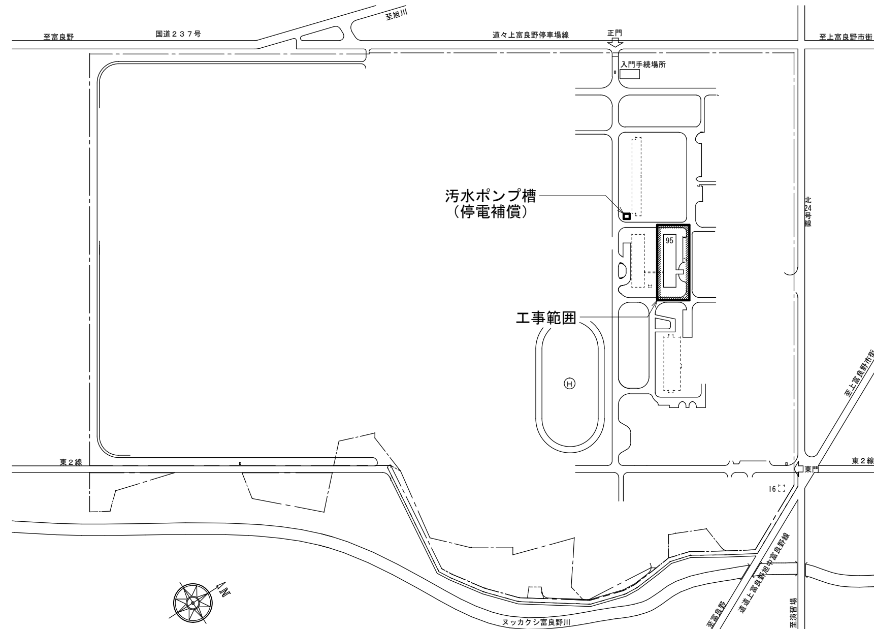
上富良野駐屯地配置図 S=1:5,000
