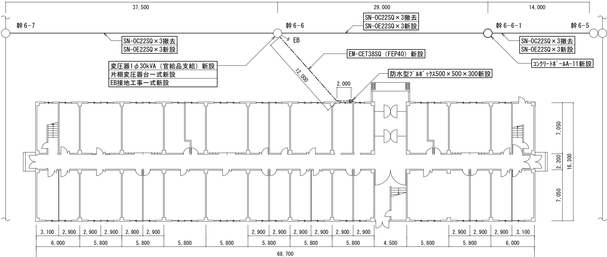
屋外配線補修図 S=1:300
