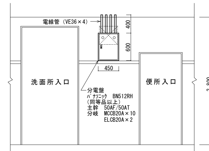
洗面所（C面）配管・機器取付詳細図 S=1:50
