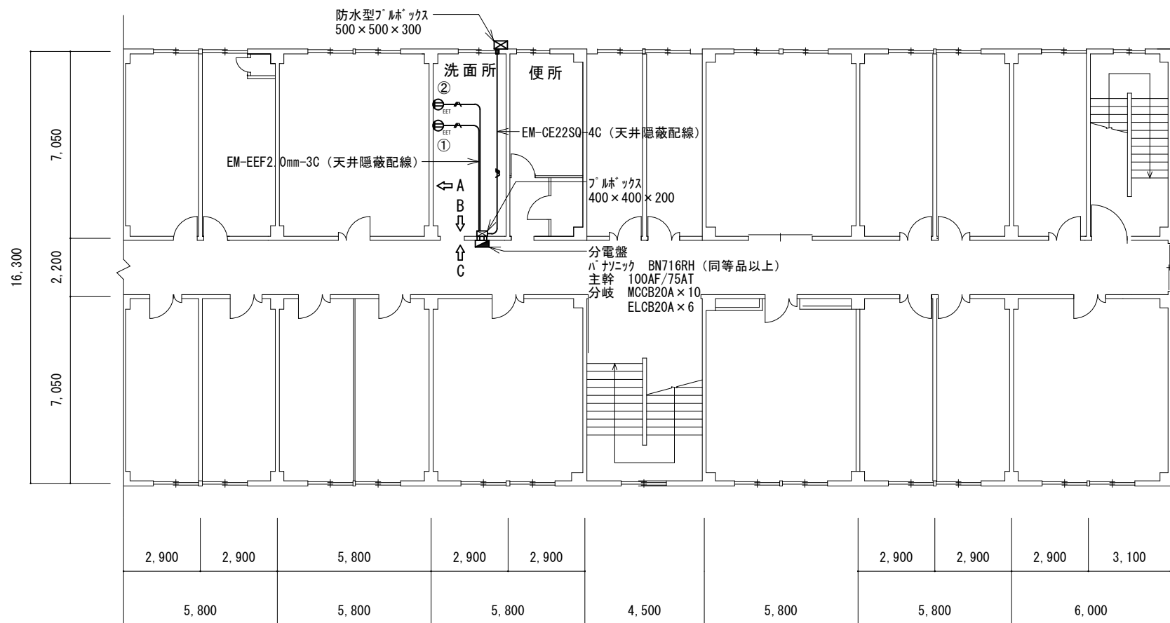
#95建物2階屋内配線補修図 S=1:200
