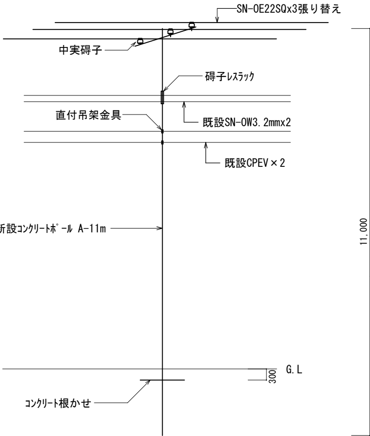
幹6-6-1号柱改修後装柱図 S=1:100
