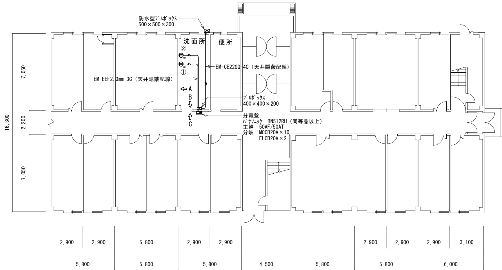
#95建物1階屋内配線補修図 S=1:200
