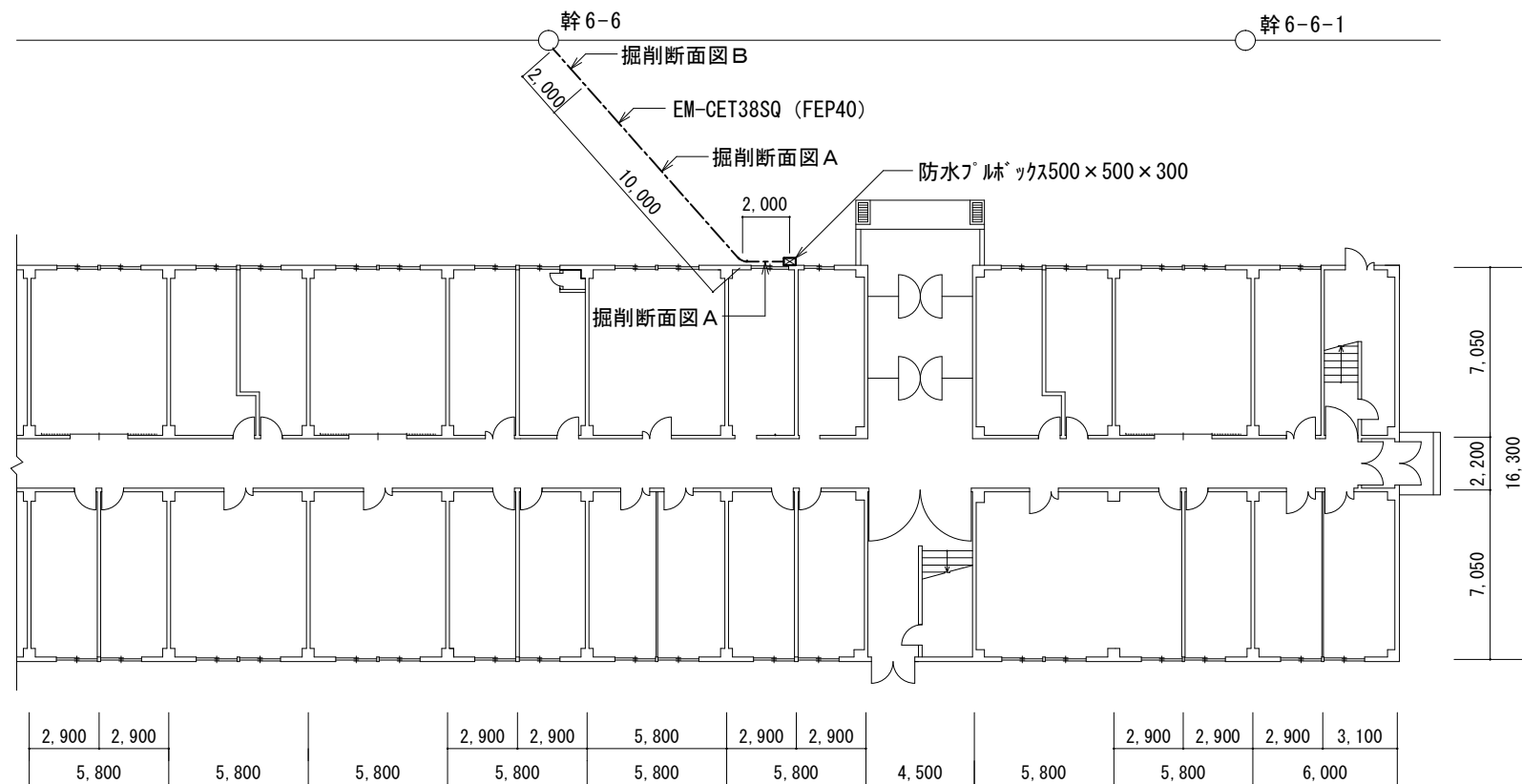
低圧埋設線敷設図 S=1:300
