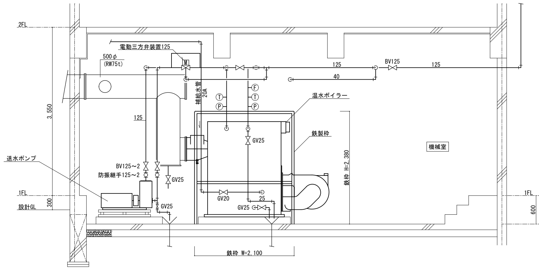
機械室断面詳細図 S=1:50
