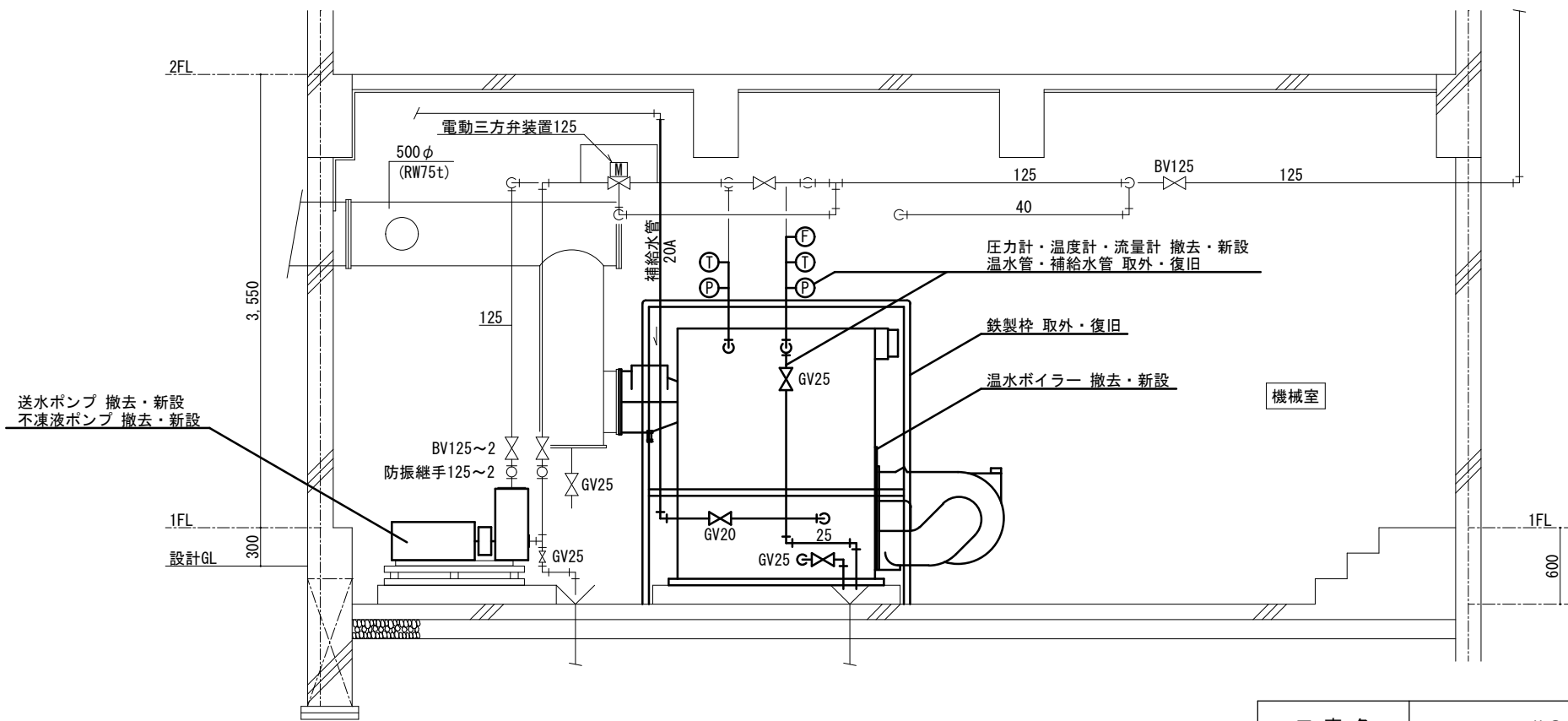
温水ボイラー交換作業箇所 S=1:50
