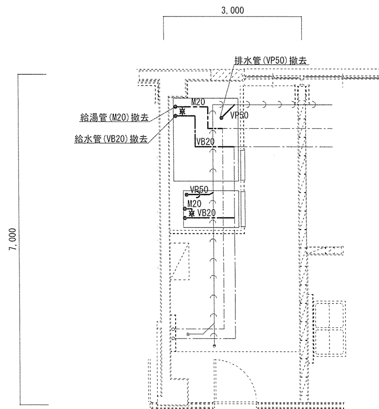
2階WAC隊舎 衛生設備配管図(撤去) S=1:80
