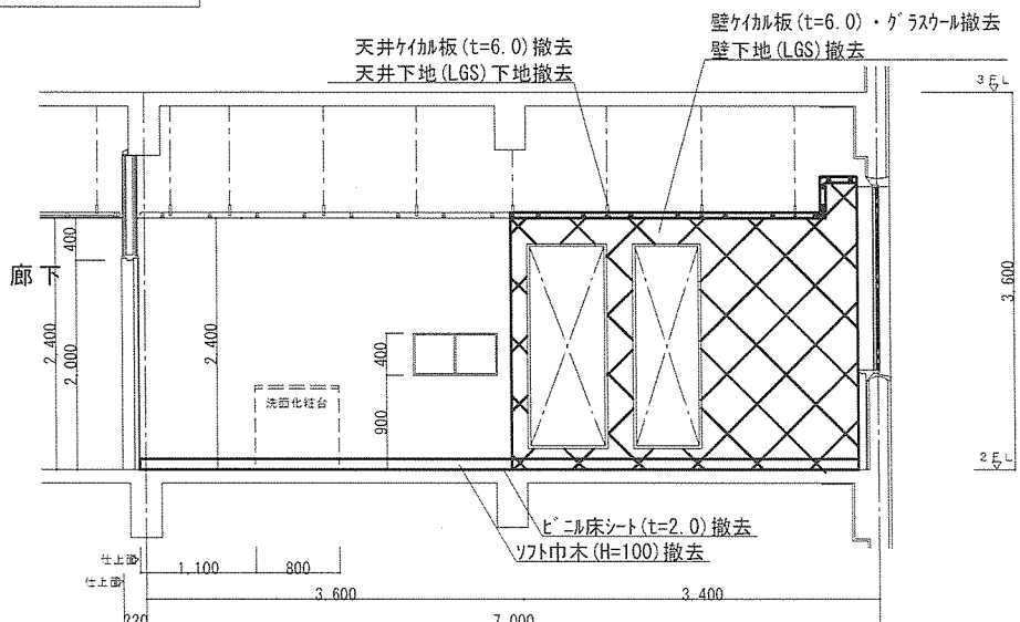
2階WAC隊舎 A面立面図(撤去) S=1:80
