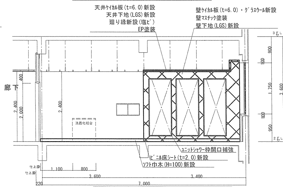
2階WAC隊舎 A面立面図(新設) S=1:80
