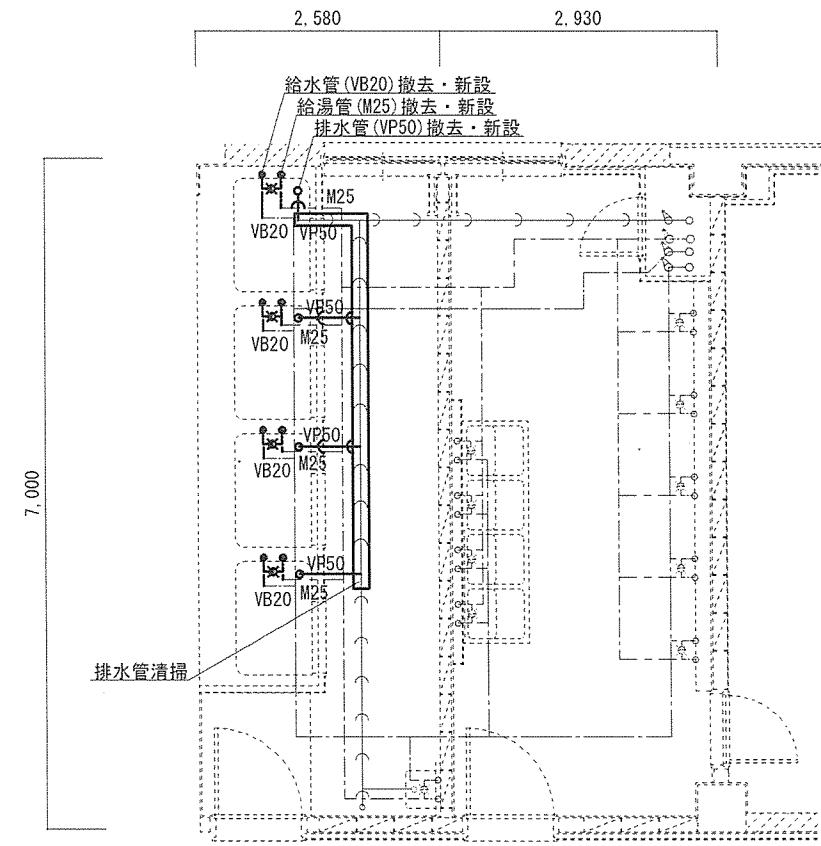
3・4生活隊舎 衛生設備配管図 S=1:80
