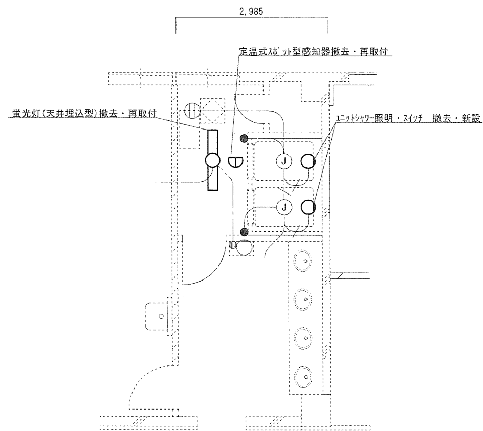
1・2階生活隊舎 電気設備図 S=1:80
