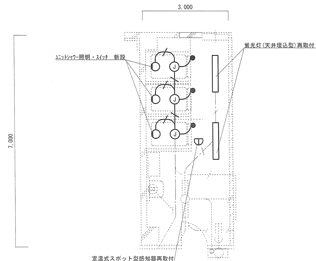
2階WAC隊舎 電気設備図(新設・再取付) S=1:80
