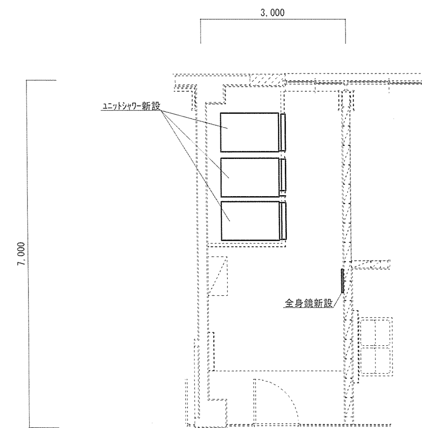
2階WAC隊舎 衛生設備図(新設) S=1:80
