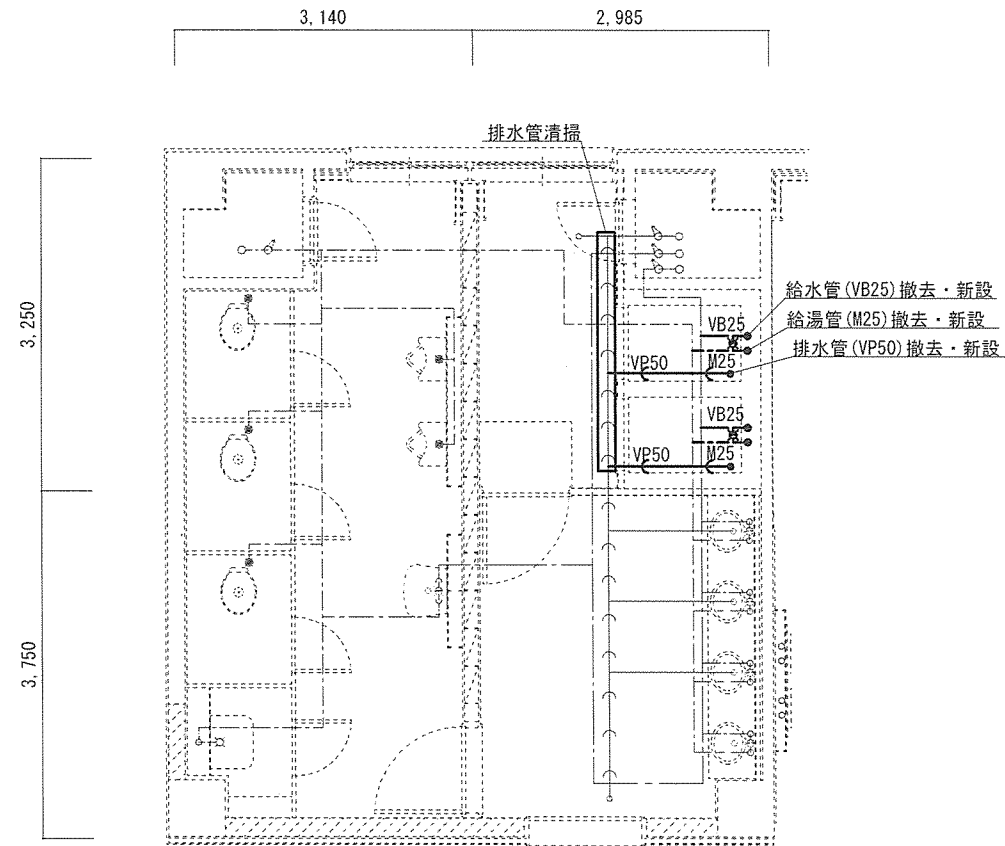
1・2階生活隊舎 衛生設備配管図 S=1:80
