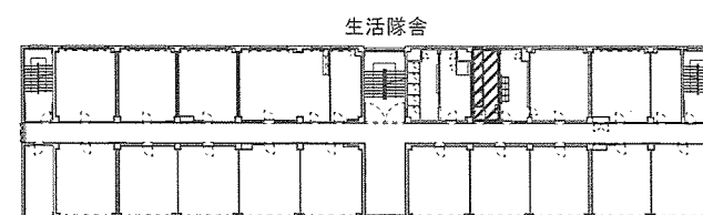
# 1 隊舎 3 階平面図
