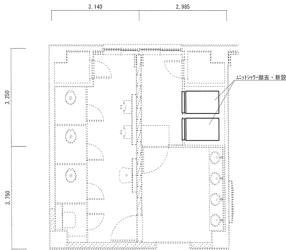
1・2階生活隊舎 衛生設備図 S=1:80
