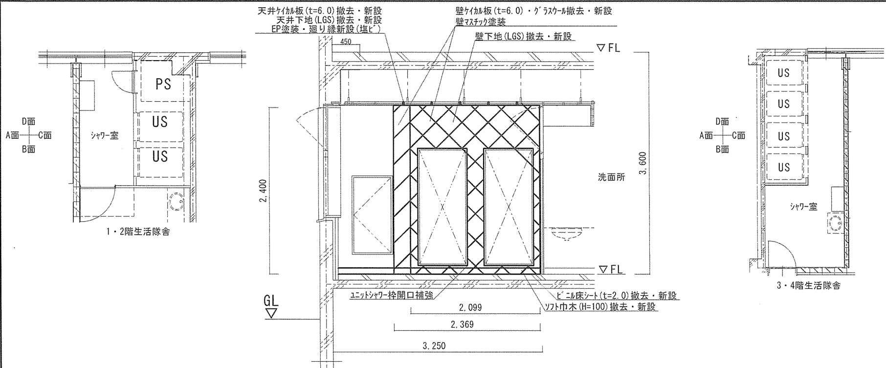
1・2階生活隊舎 C面立面図 S=1:60
