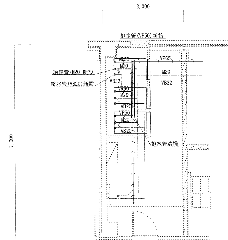
2階WAC隊舎 衛生設備配管図(新設) S=1:80
