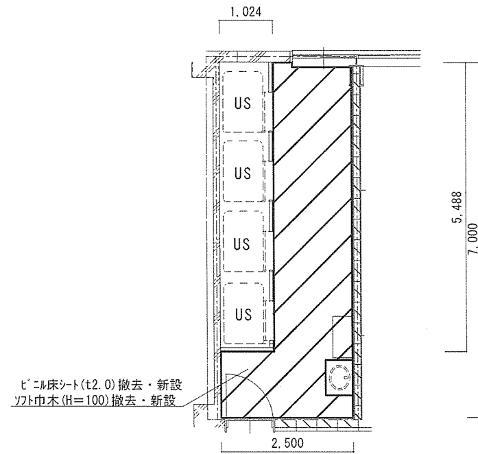
3・4階生活隊舎 床平面図 S=1:100
