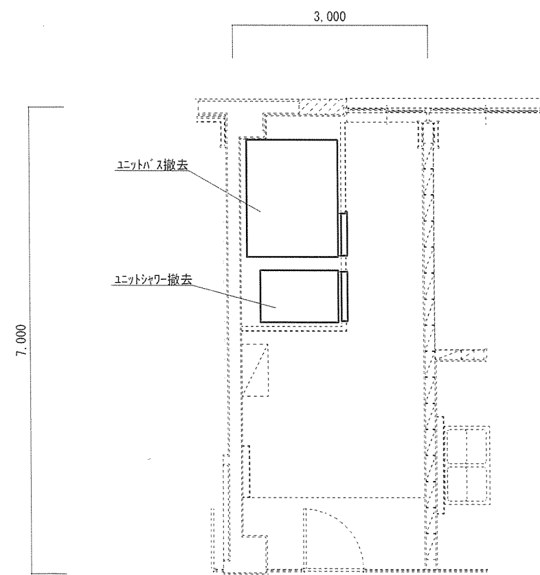
2階WAC隊舎 衛生設備図(撤去) S=1:80
