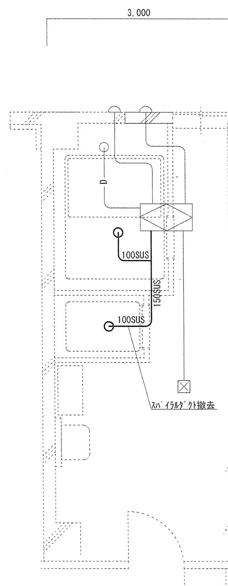
2階WAC隊舎 換気設備図(撤去) S=1:80
