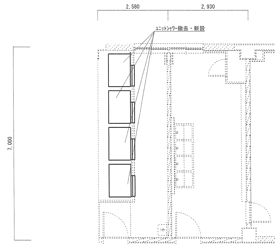
3・4階生活隊舎 衛生設備図 S=1:80
