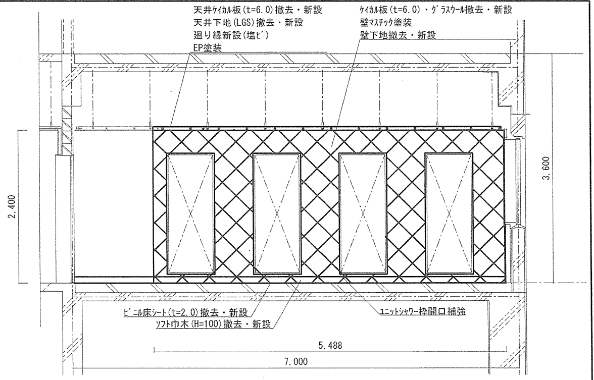
3・4階生活隊舎 A面立面図 S=1:60
