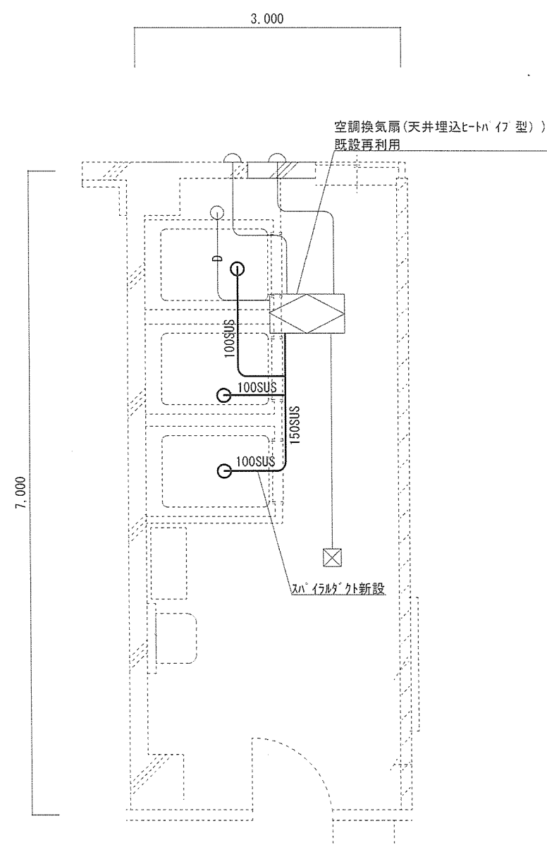
2階WAC隊舎 換気設備図(新設) S=1:80
