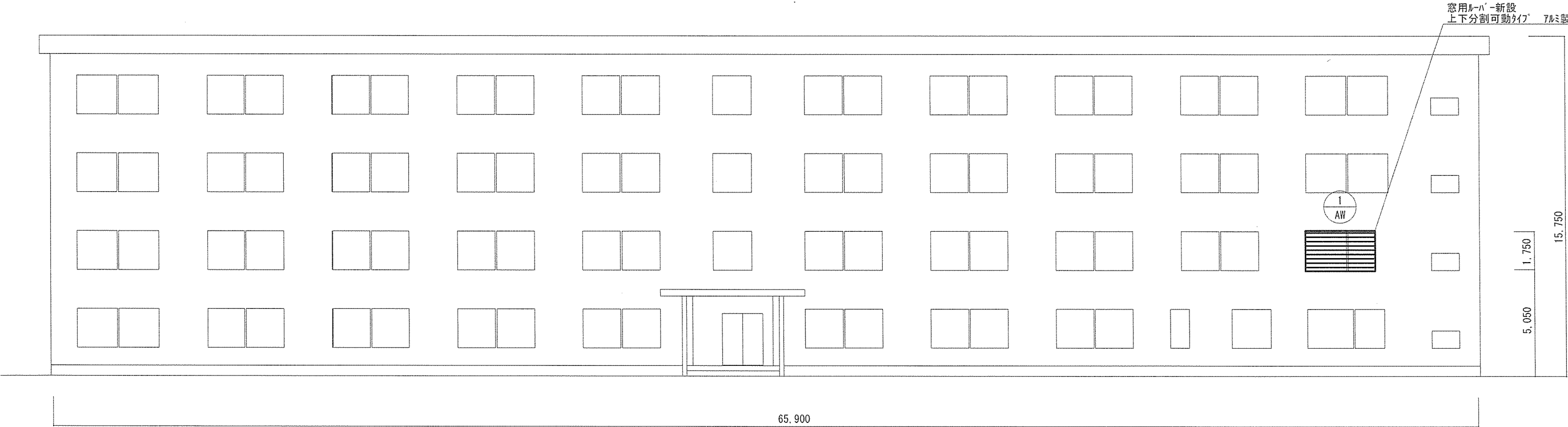
生活隊舎 北側立面図 S=1:200
