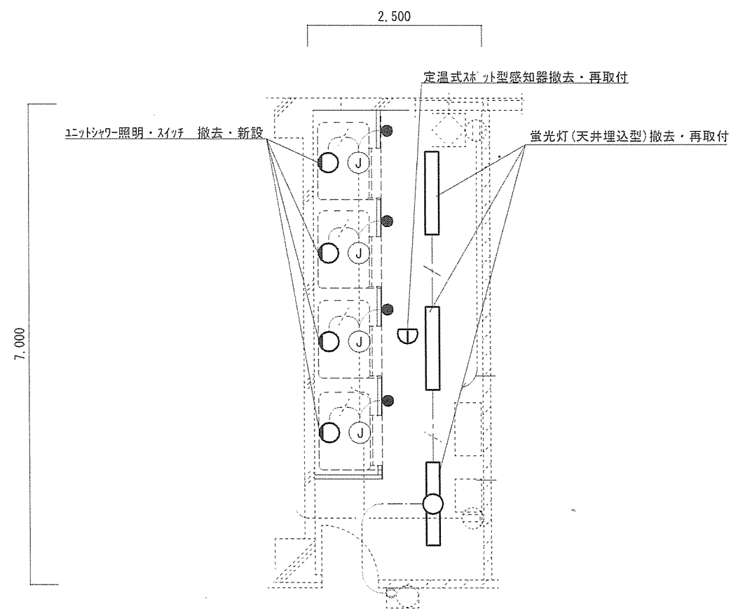
3・4階生活隊舎 電気設備図 S=1:80
