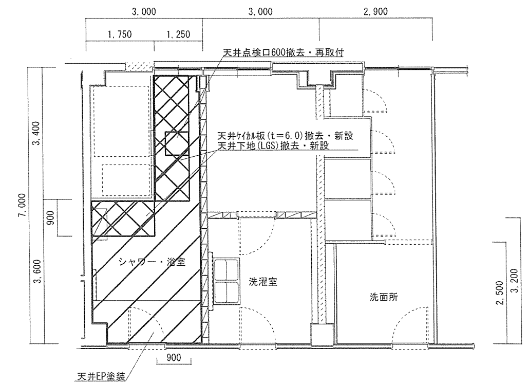
2階WAC隊舎 天井伏図 S=1:100
