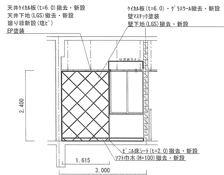
2階WAC隊舎 D面立面図 S=1:80
