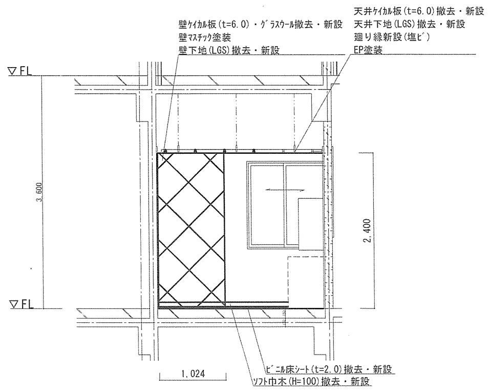
3・4階生活隊舎 D面立面図 S=1:60
