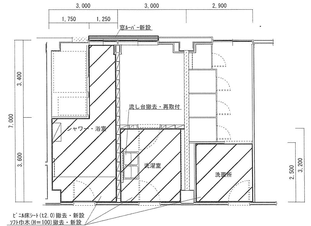
2階WAC隊舎 床平面図 S=1:100
