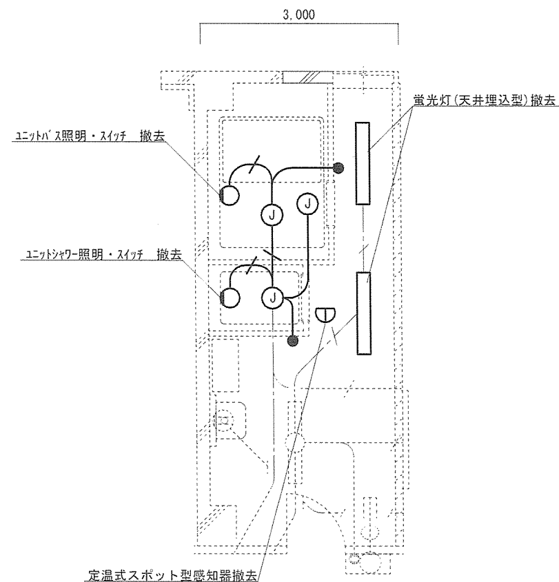
2階WAC隊舎 電気設備図(撤去) S=1:80
