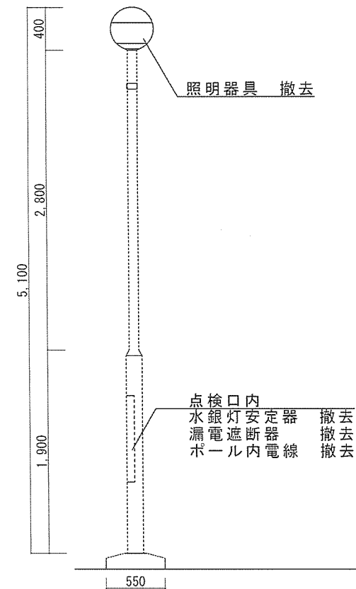
街路灯②③ 姿図 S = 1/50
