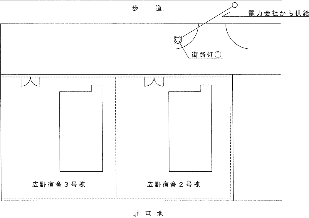
街路灯 配置図 S = 1/150
