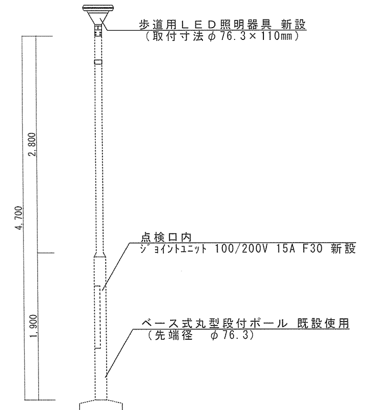
補修後
