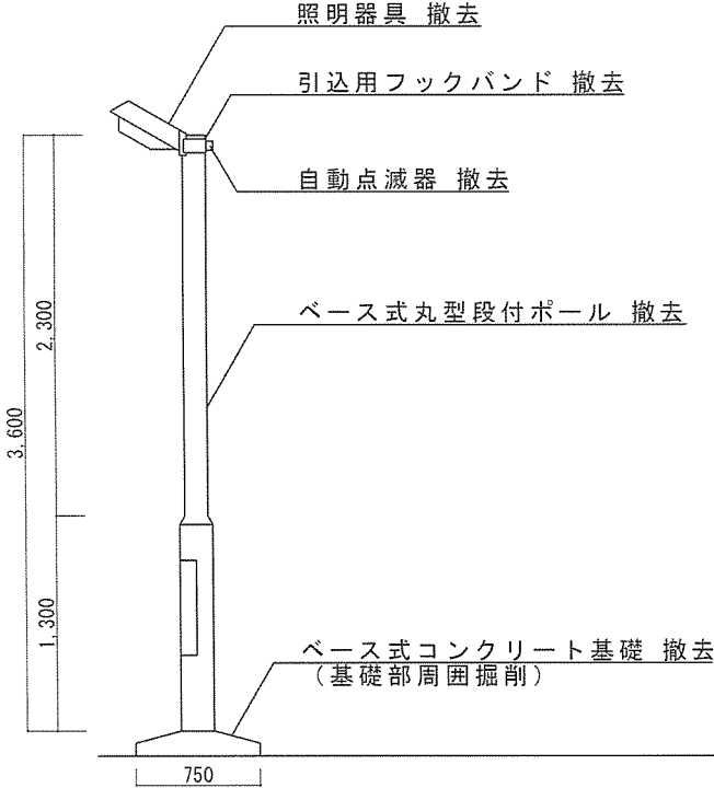
補修前
