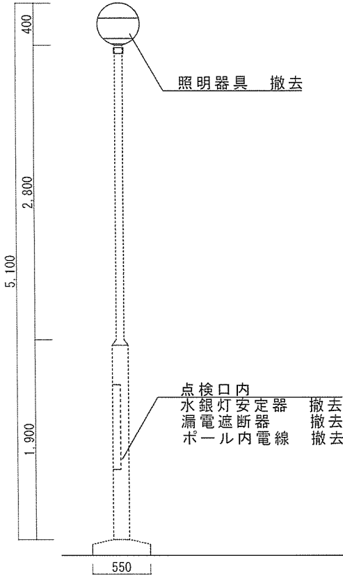
街路灯④ 姿図 S = 1/50
