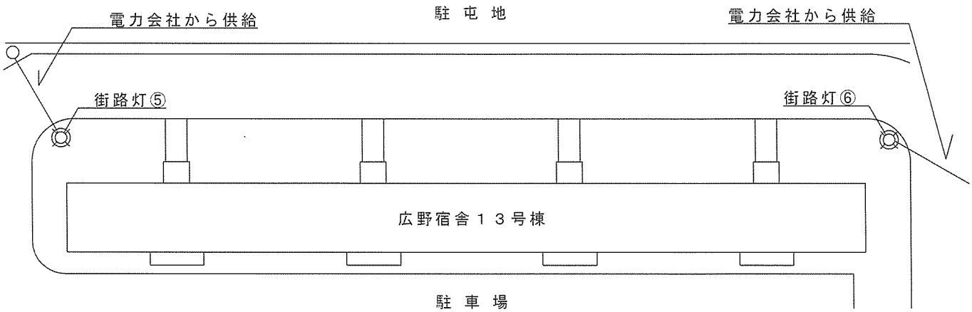
街路灯 配置図 S = 1/500
