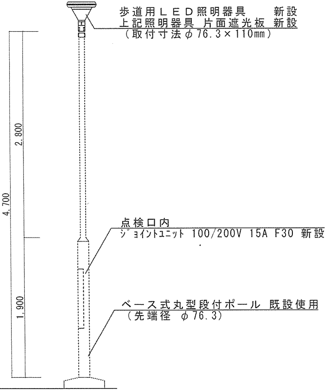
補修後
