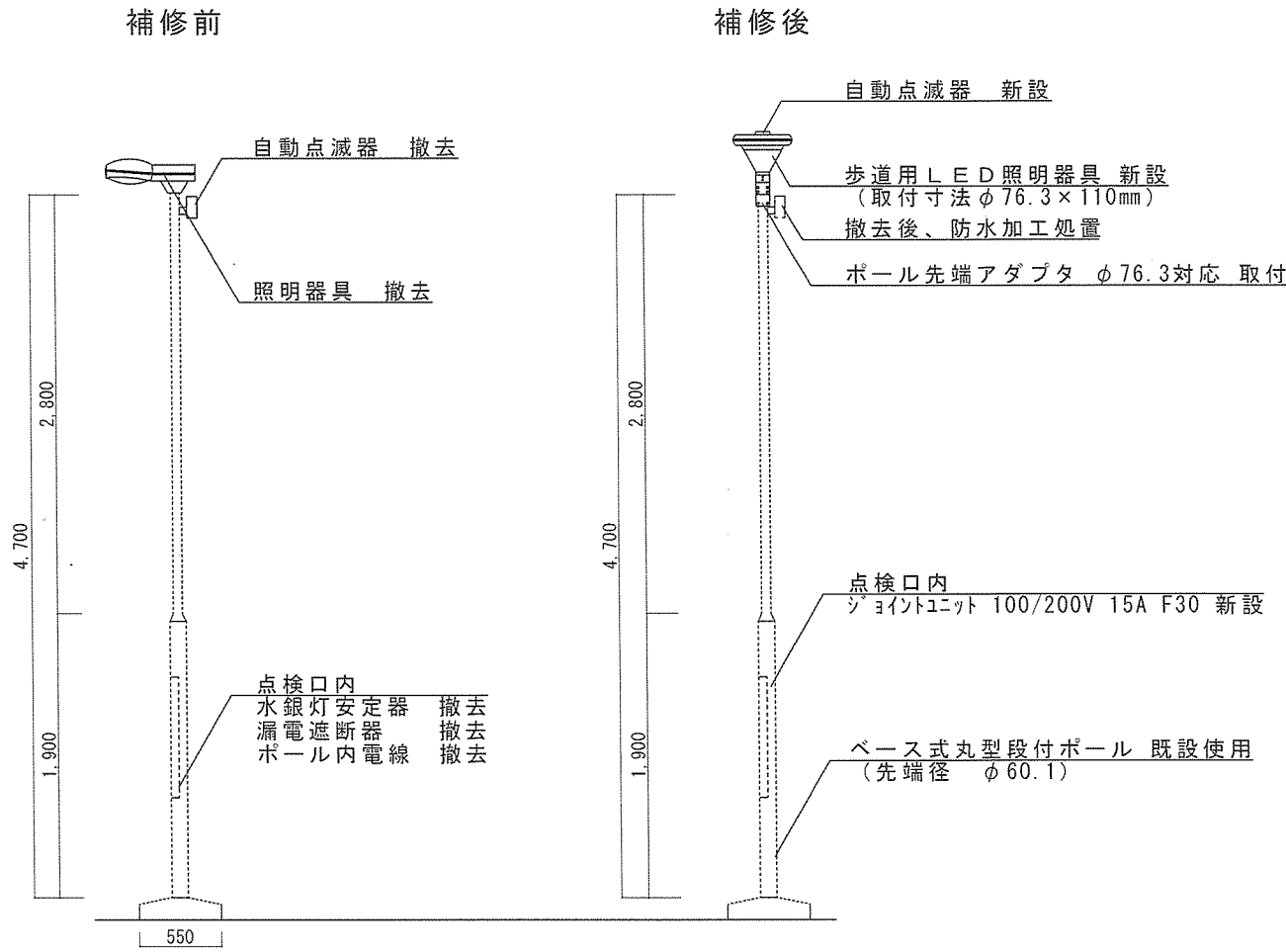
街路灯⑤⑥ 姿図 S = 1/50
