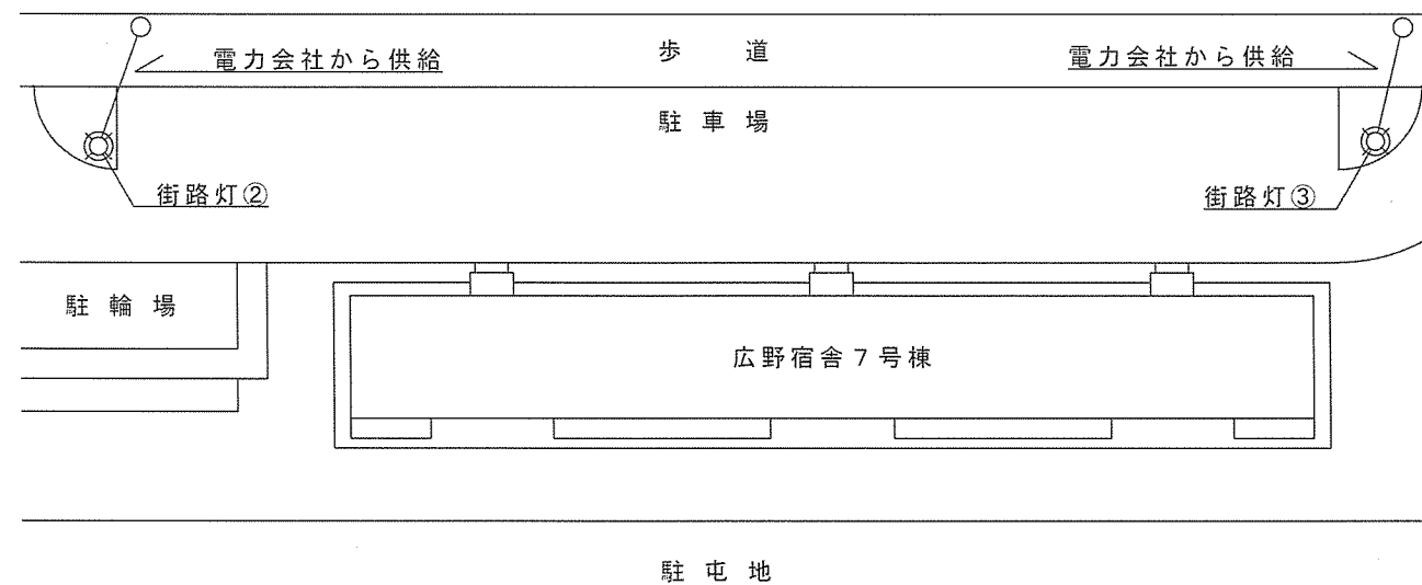
街路灯 配置図 S = 1/300
