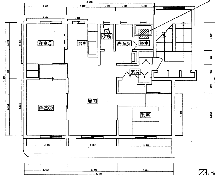
6号棟平面図 S=1/100
