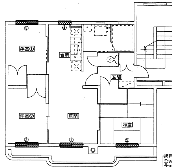
5号棟平面図 S=1/100
