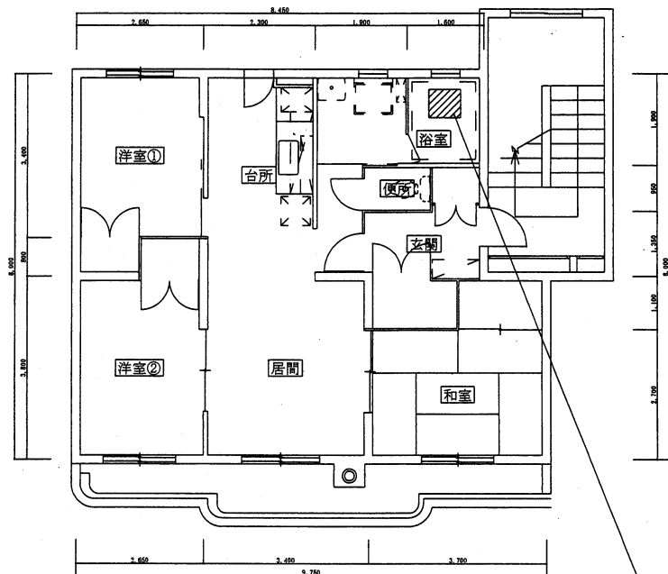
5号棟平面図 S=1/100
