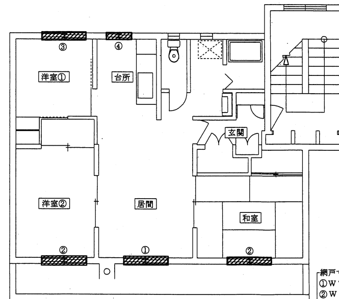
6号棟平面図 S=1/100
