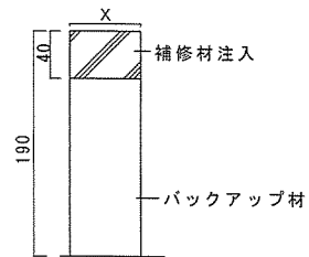
クラック補修標準図 S=1 : X
