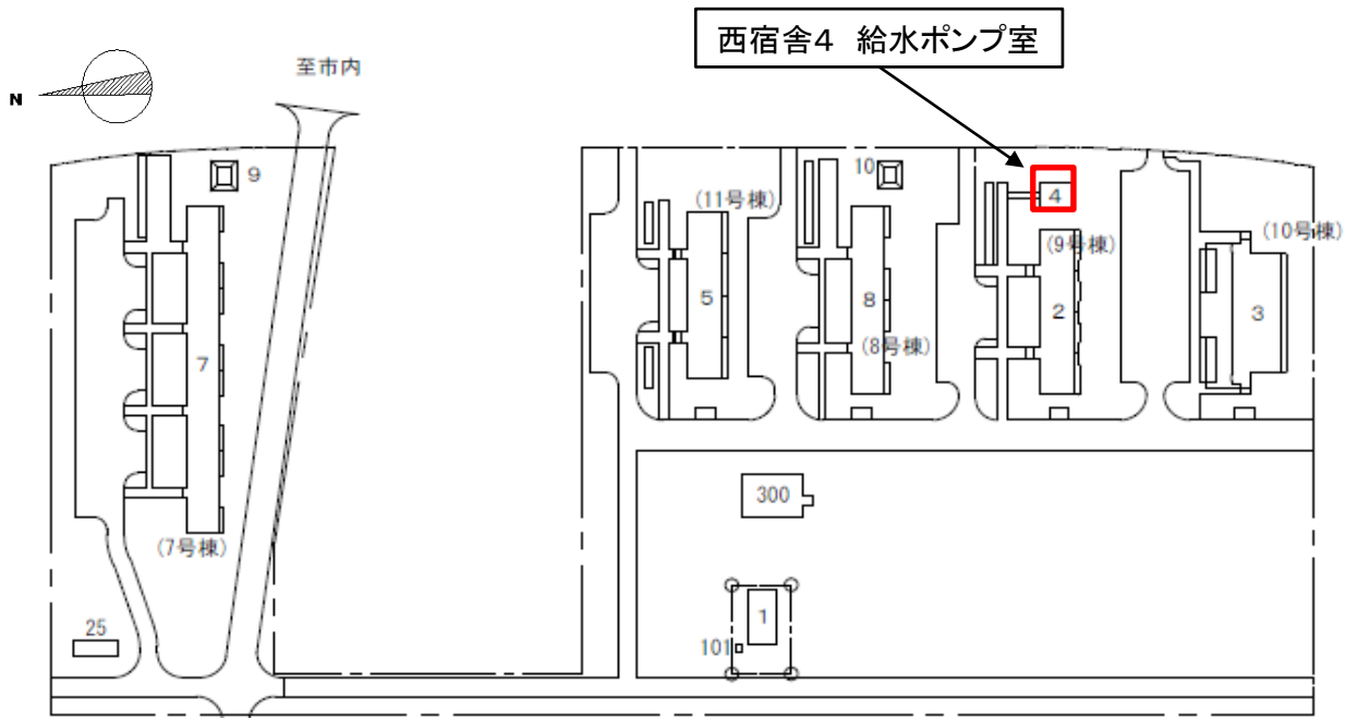
宿 舎 配 置 図 1/2,000
