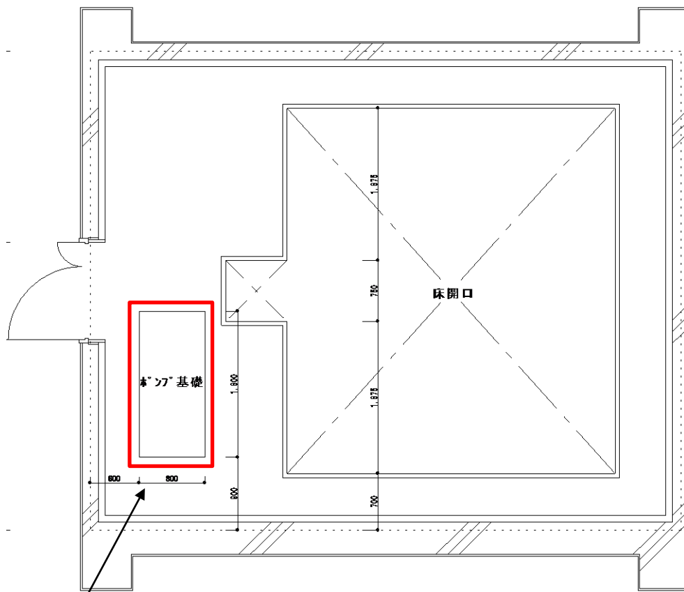
自動給水装置更新箇所
