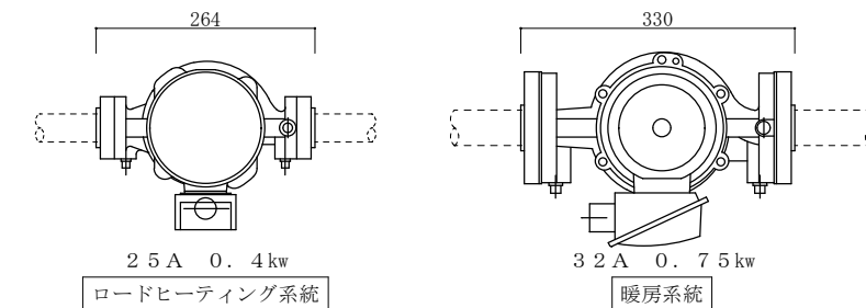
循環ポンプ標準図 S=1:10
