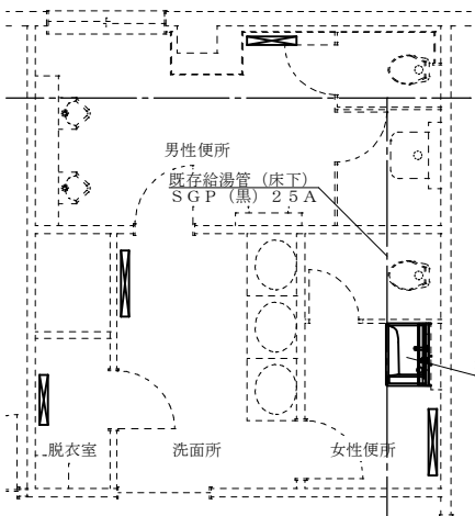
水回り更新平面図 S=1:100
