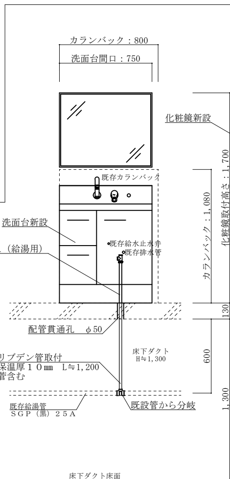
洗面化粧台更新標準図 S=1:30
