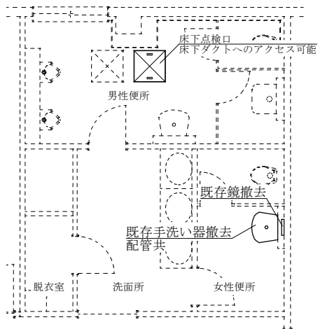
水回り既存平面図 S=1:100
