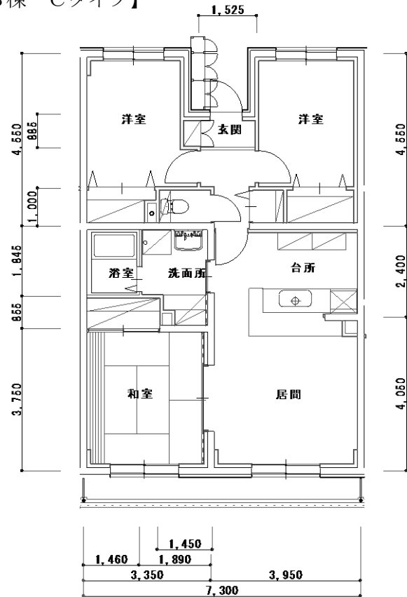
【本町 B棟 Cタイプ】
