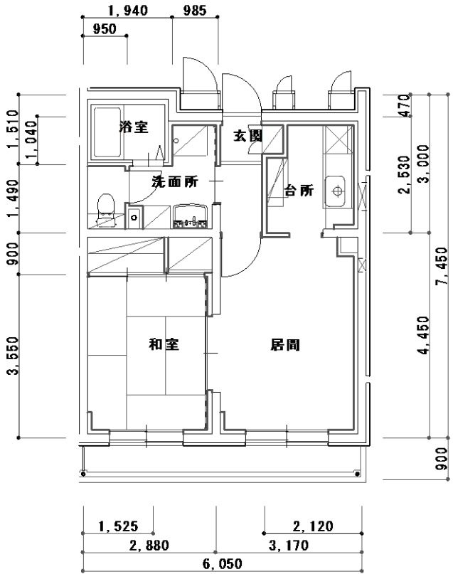
【本町 B棟 単bタイプ】
