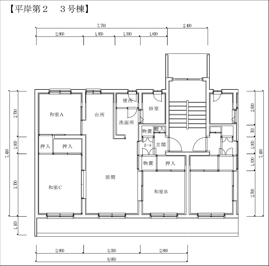
④ 平岸第2 宿舍平面図
