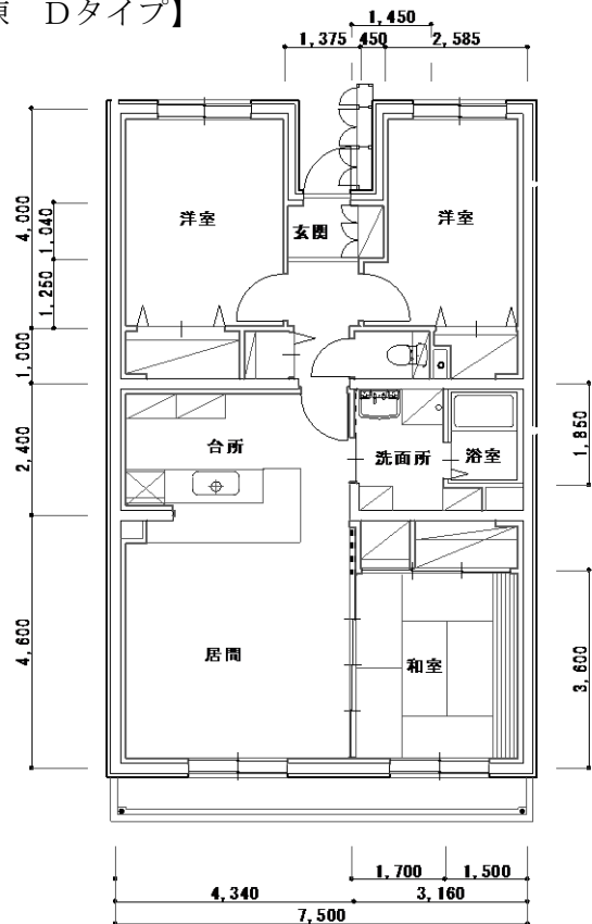
【本町 B棟 Dタイプ】
