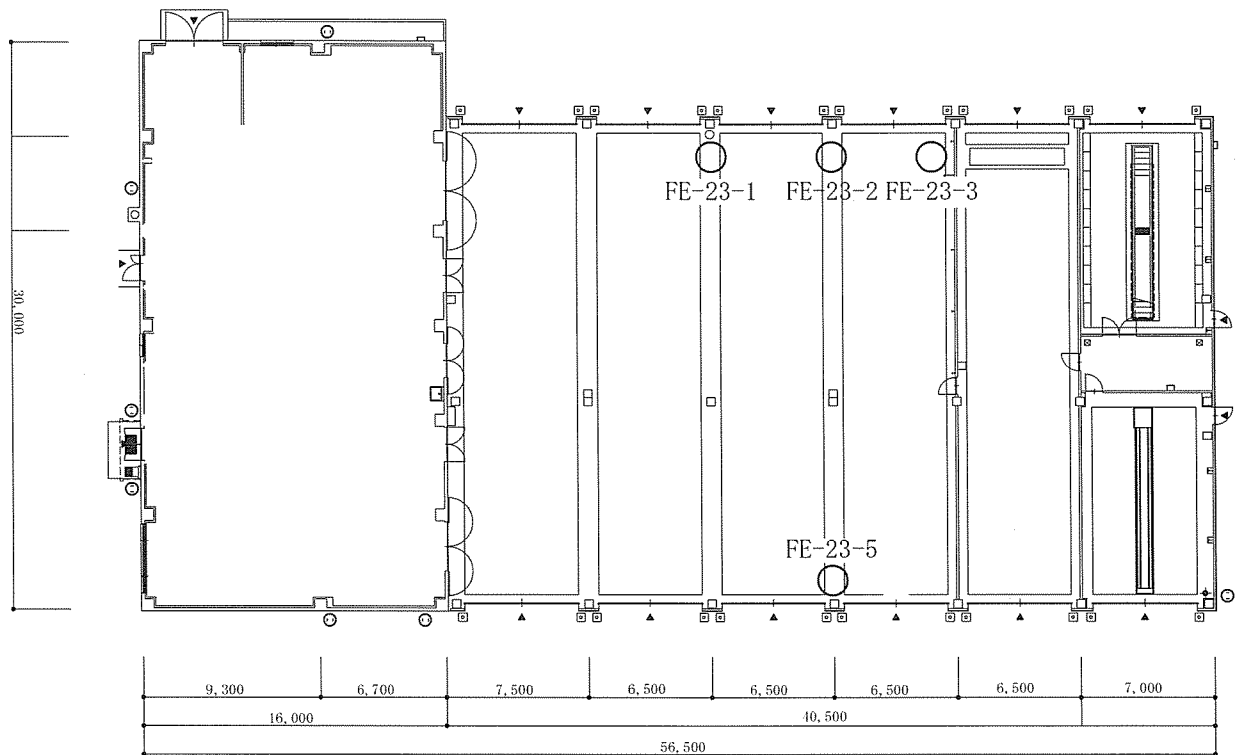
#29整備工場 平面図 S=1:400
