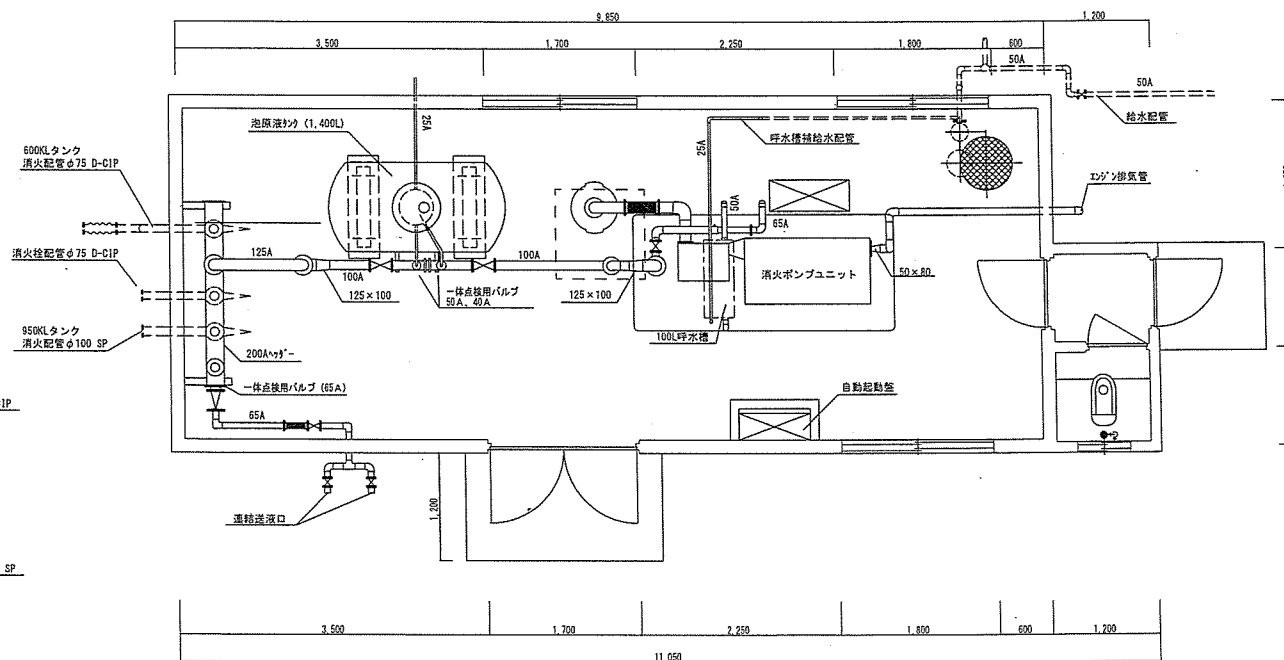
#41建物平面図 S=1/60
