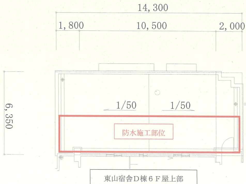
図2－防水施工部位
