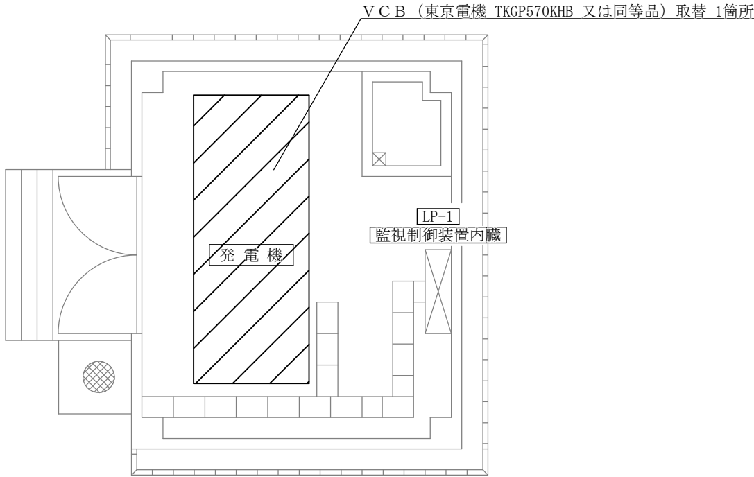
172号建物平面図 S=1/100
