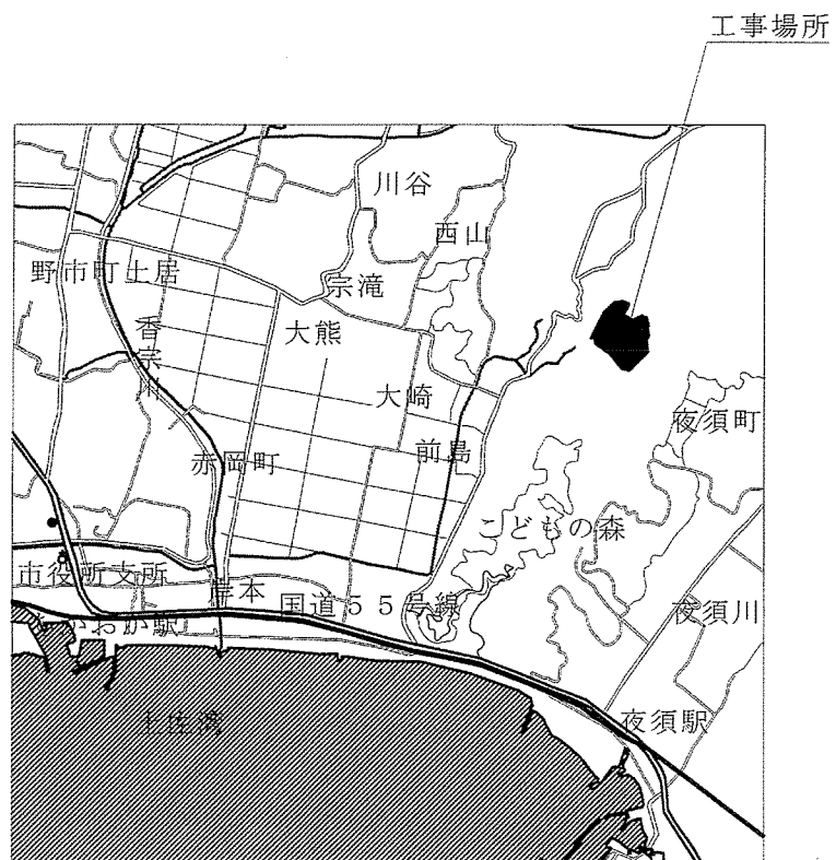
高知駐屯地(第1営舎地区)案内図 S = 1 / X
