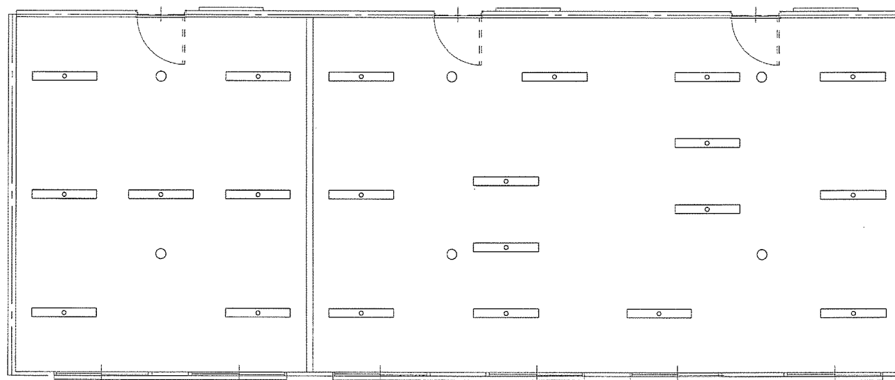
居室 (1スパン)・居室 (2スパン) 内 電灯設備詳細図
