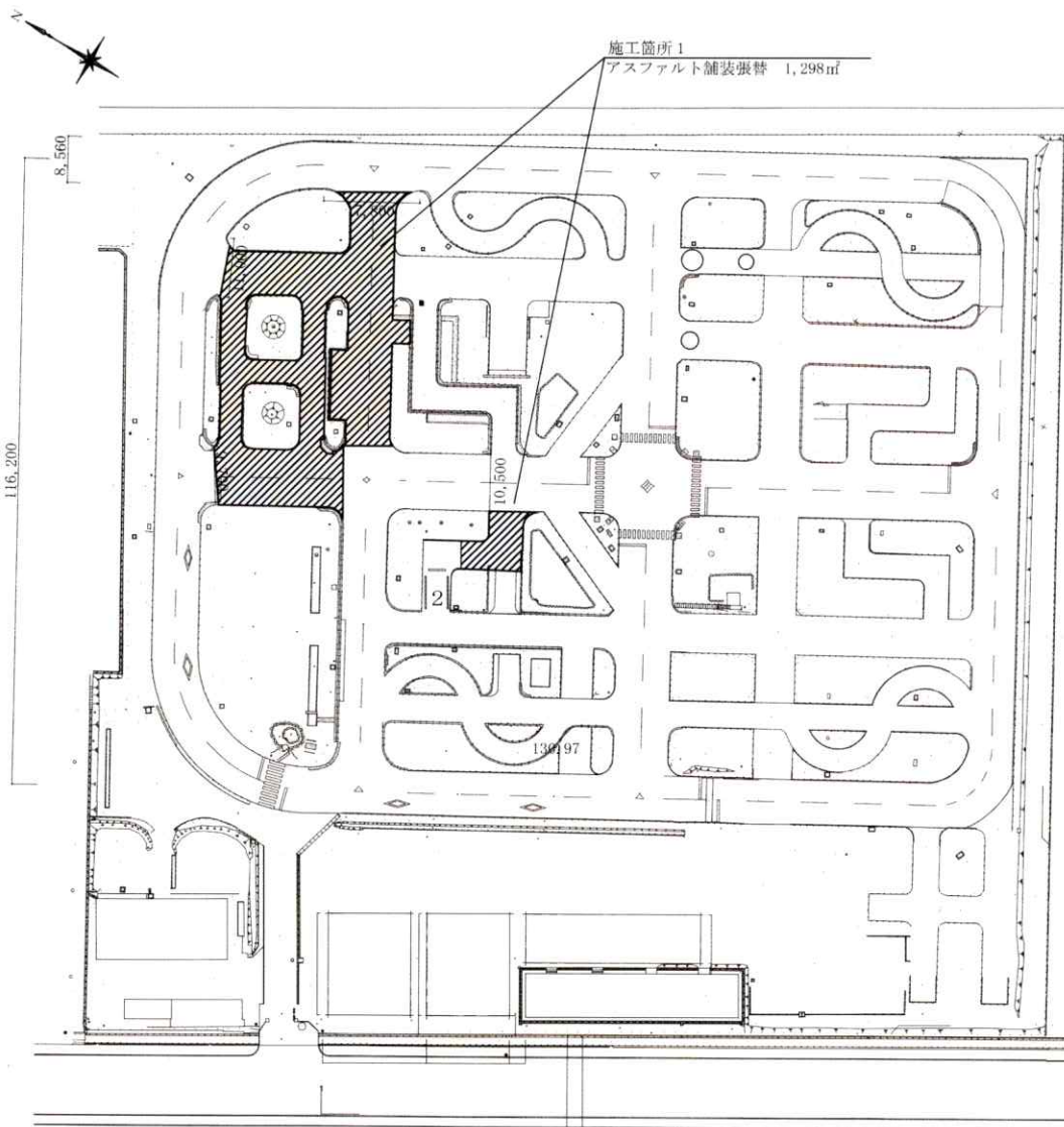
自動車教習場配置図 S=1/1,000
