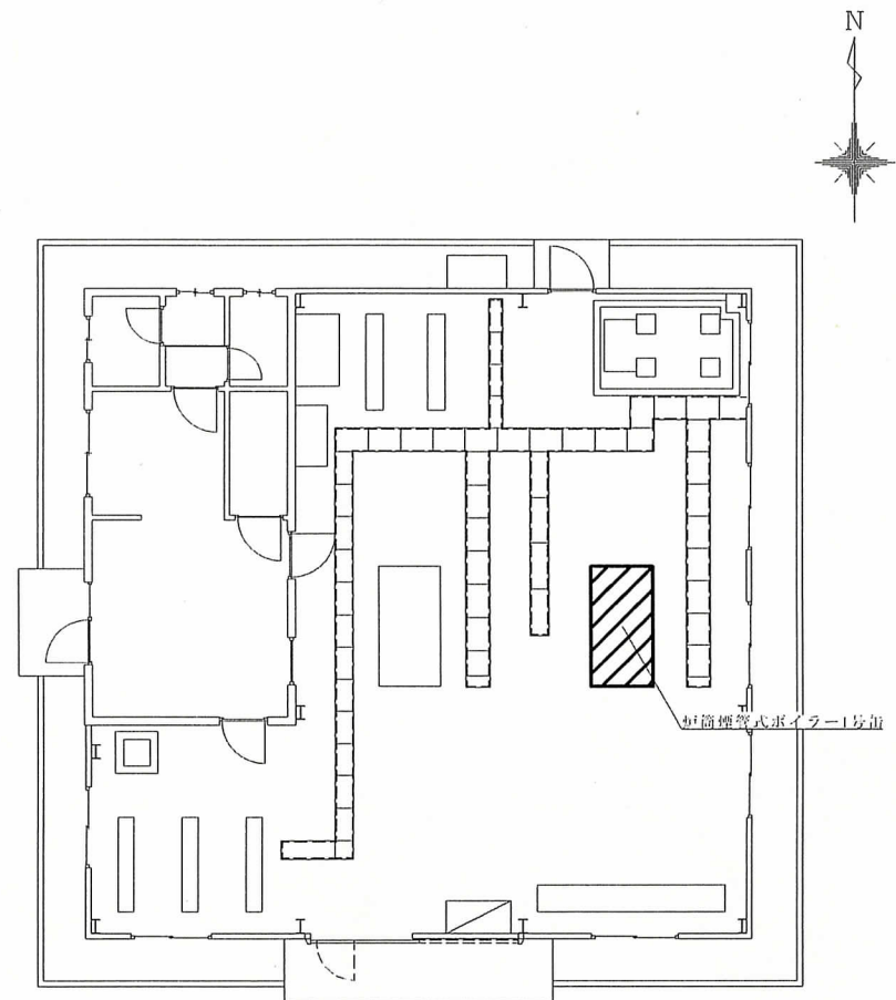
11号ボイラー室平面図
