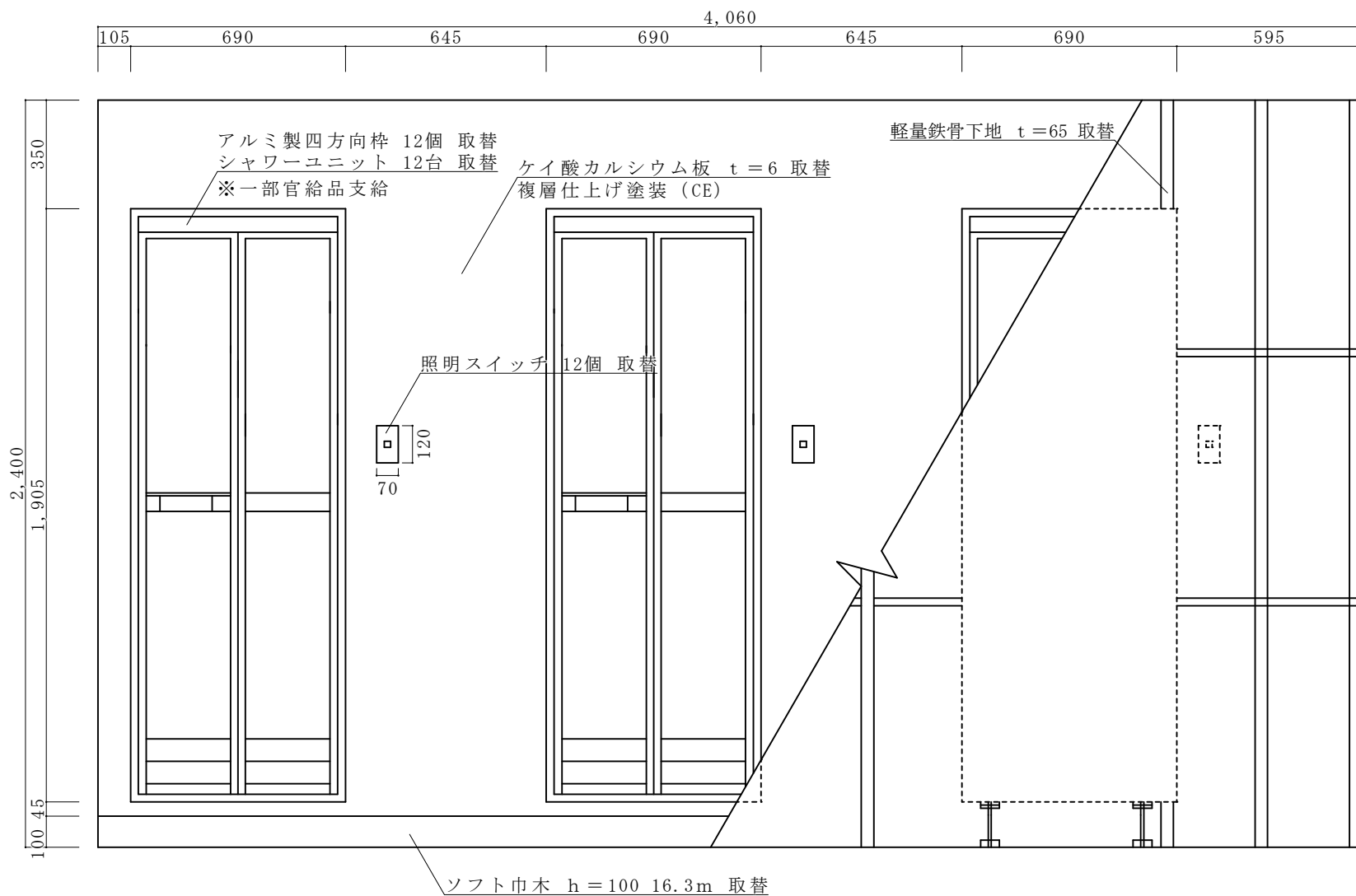
2～5階シャワー室立面図 S=1/20
