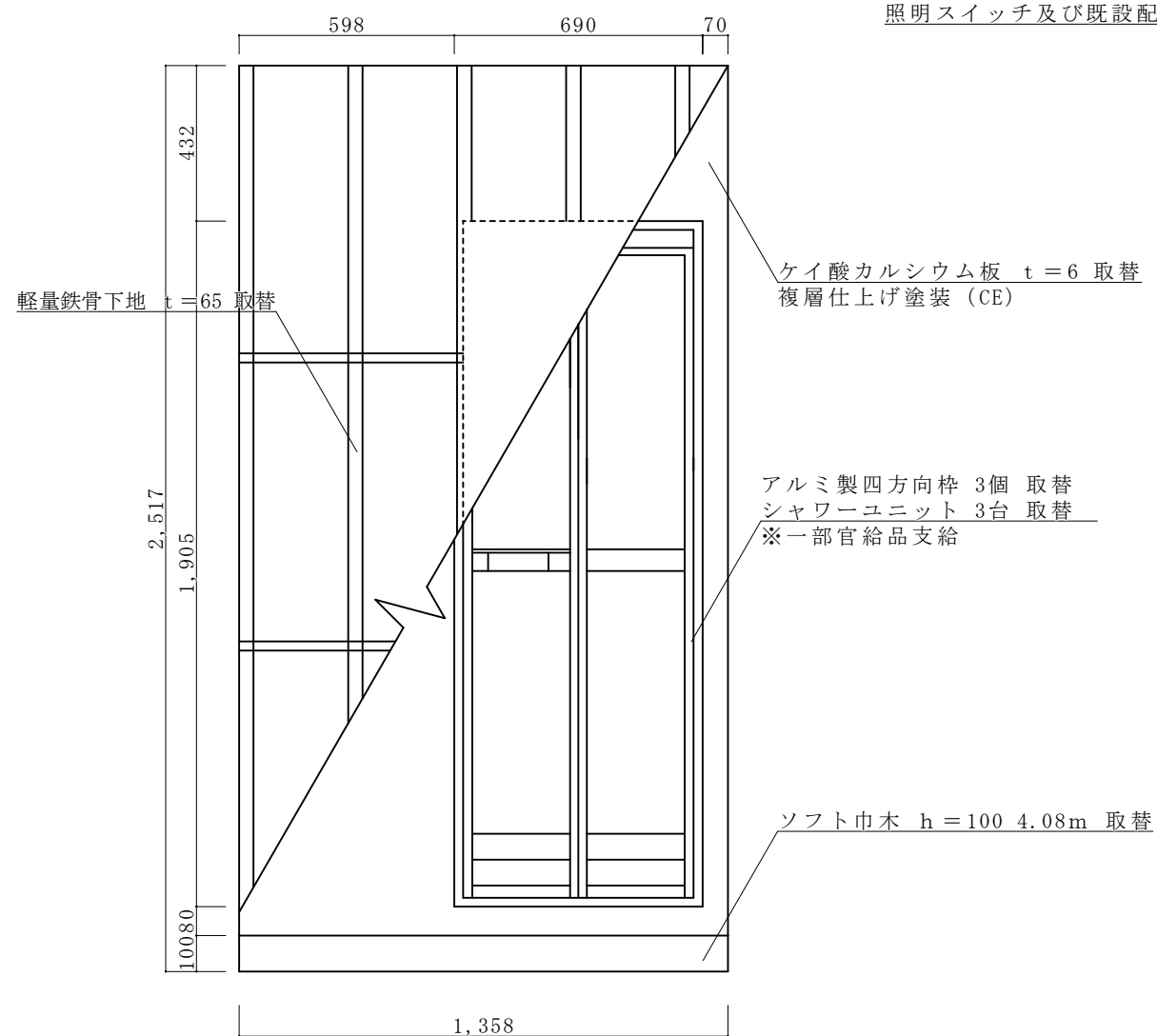
1～3階シャワー室立面図 S=1/20
