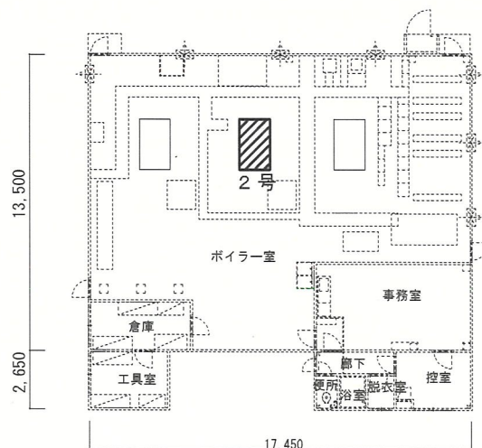
15号建物平面図 S=1/300
