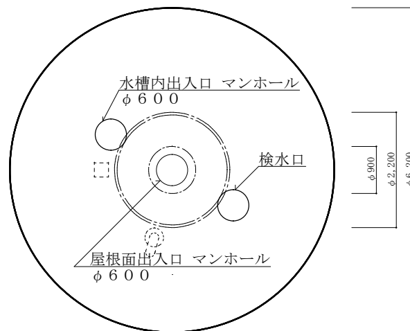
B-B平面図
