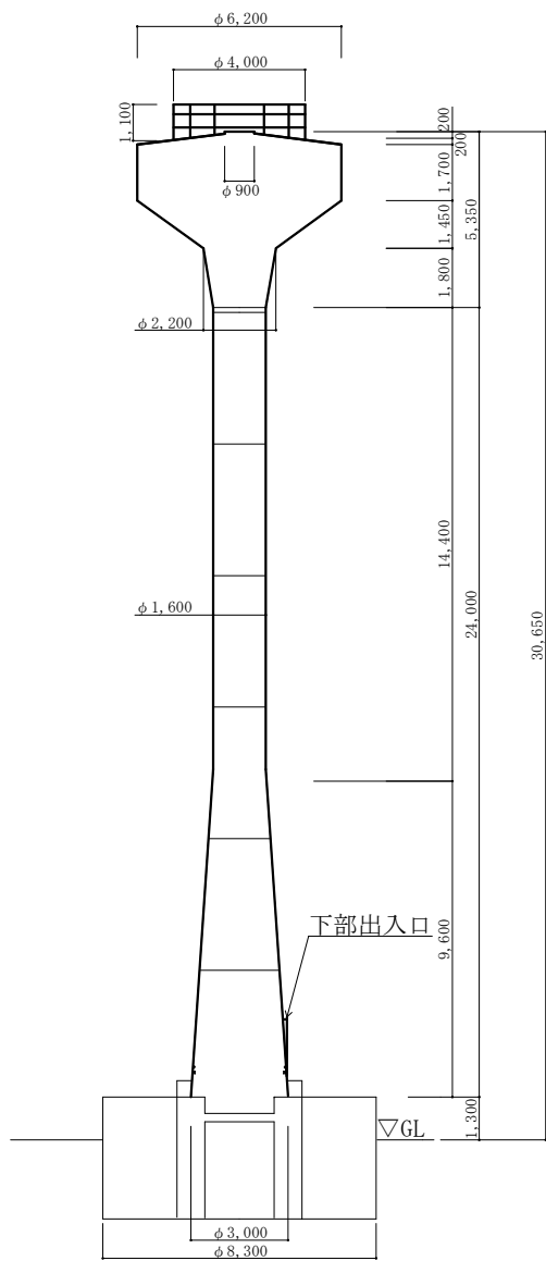
高架水槽立面図 S=1/250
