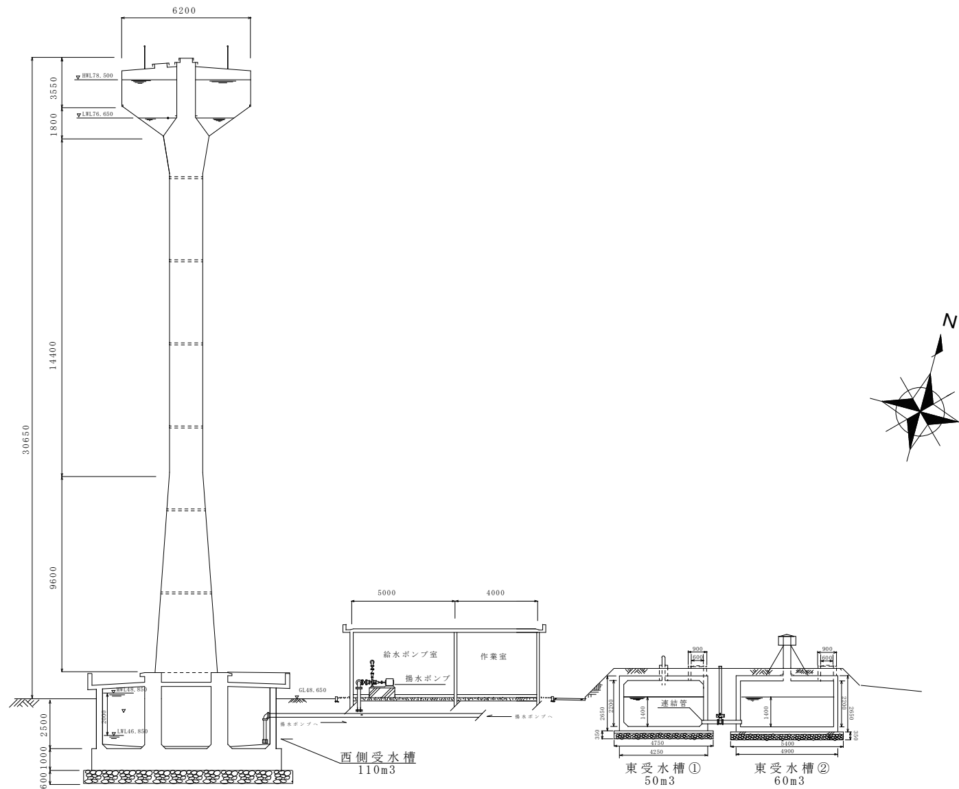
給水施設配置図 S=1/X
