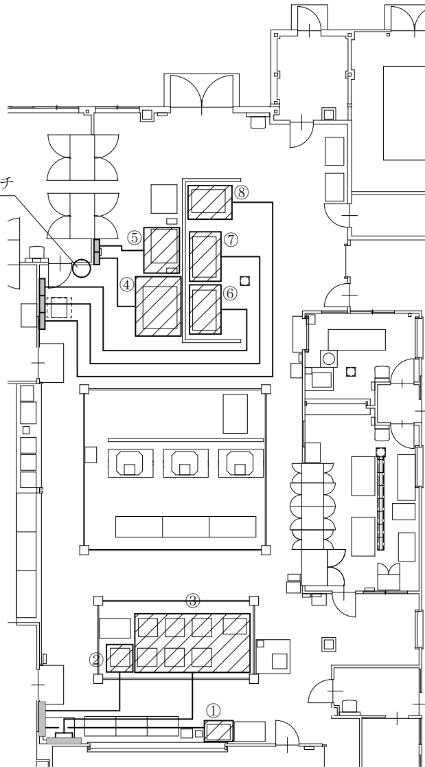
248号建物厨房部分平面図 S=1/200
