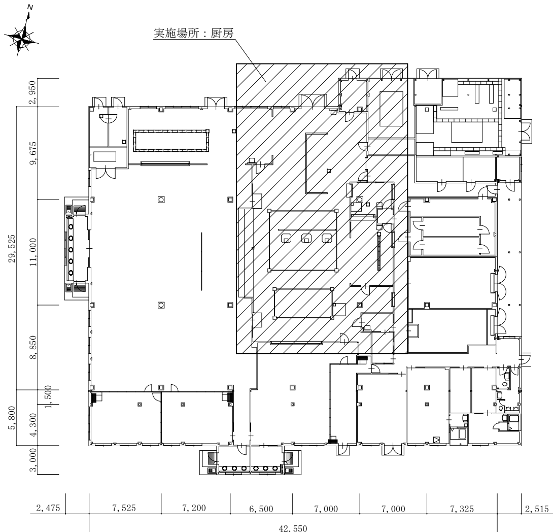
248号建物平面図 S=1/400
