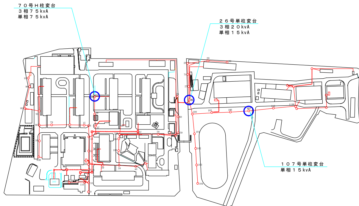
千僧駐屯地高压配線図 S=1/N
