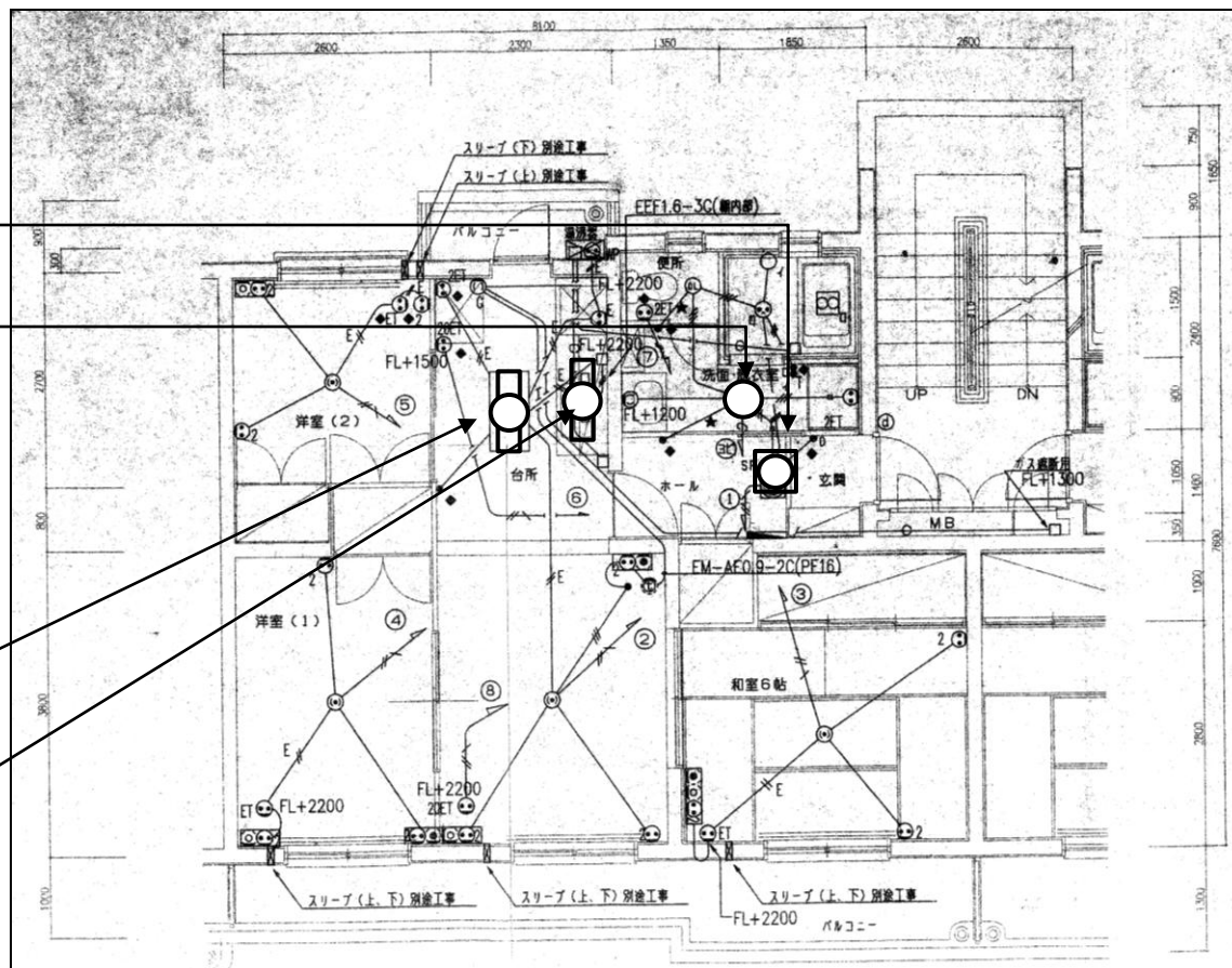
標準図 1
