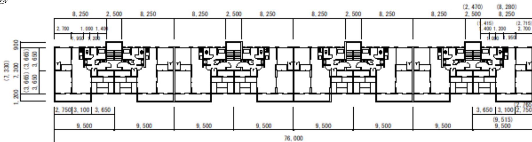
平面図（1階～5階）
