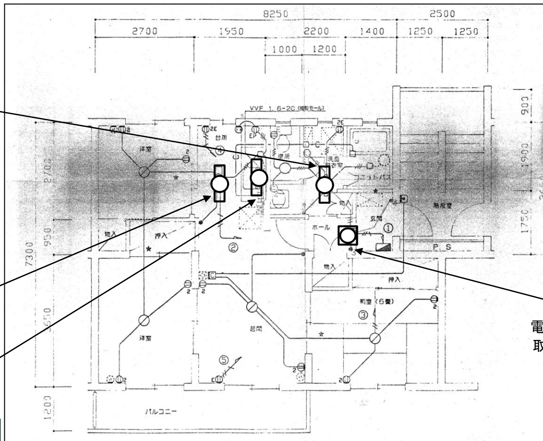
標準図
