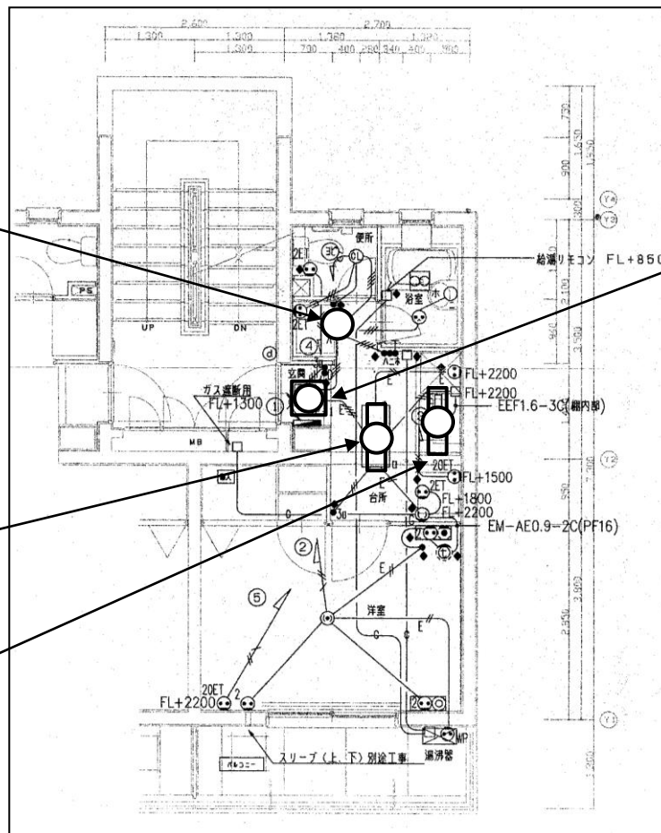
標準図 2
