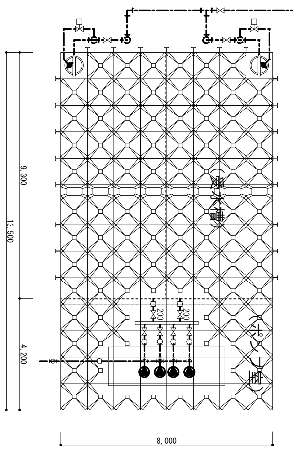
山本-2 (平面図)
