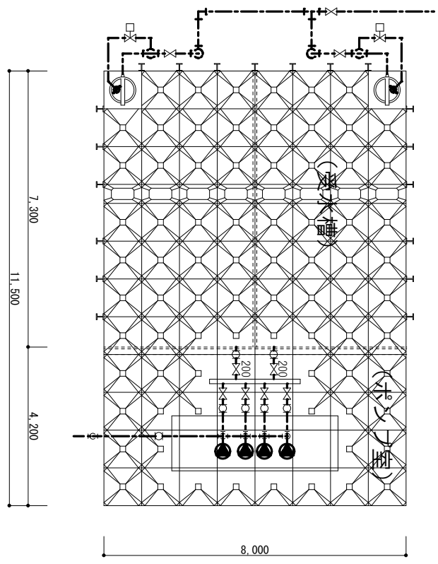
山本-1 (平面図)
