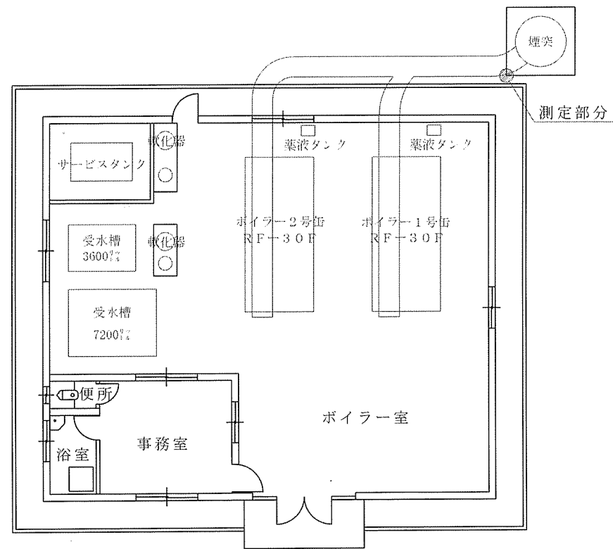
ボイラー室平面図 縮尺：1/150
