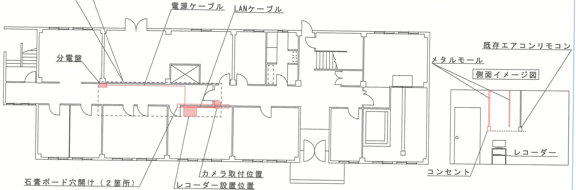
23号生活隊舎1階平面図
