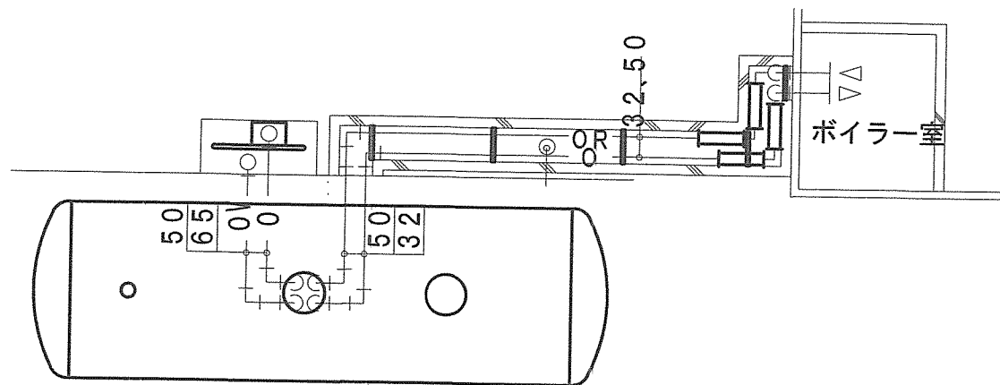
地下燃料タンク配置詳細図 S=1:X
