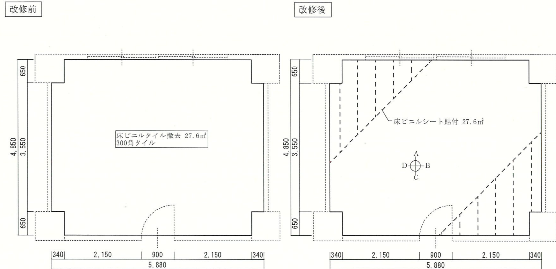
床改修参考図 S=1/50
