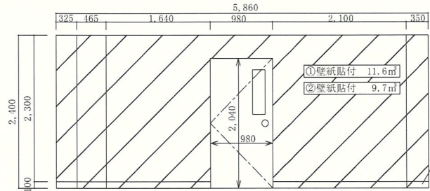
壁改修参考図 S=1/40
