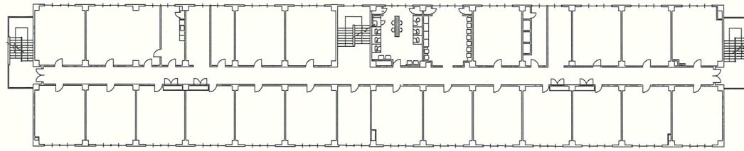
111号建物平面図 (標準) S=1/300
