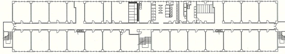
4号建物平面図 (標準) S=1/300
