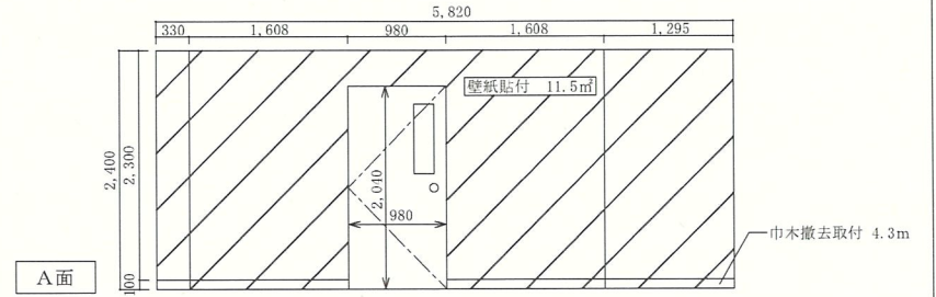
壁改修参考図 S=1/40
