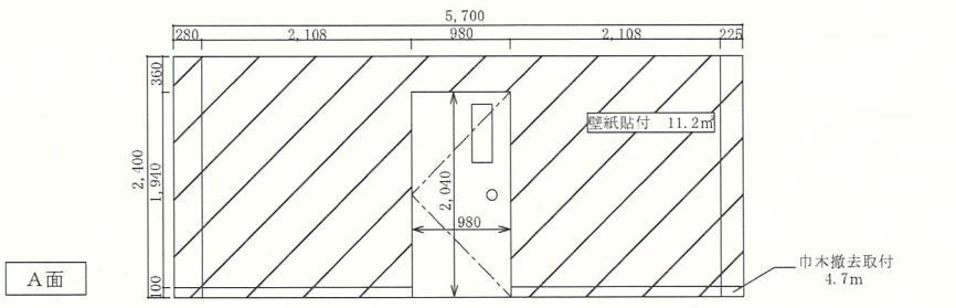
壁改修参考図 S=1/40
