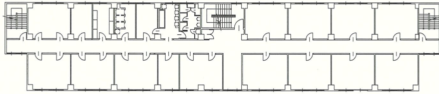
116号建物平面図 (標準) S=1/250
