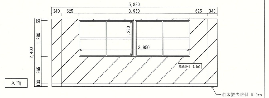
壁改修参考図 S=1/40
