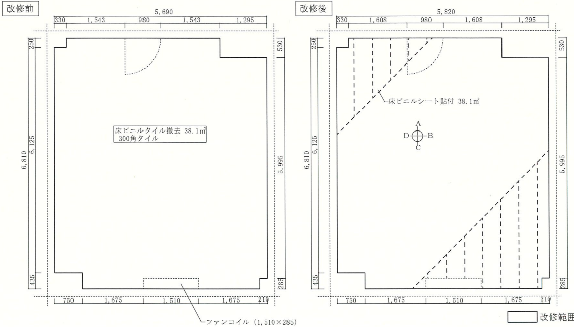
床改修参考図 S=1/50
