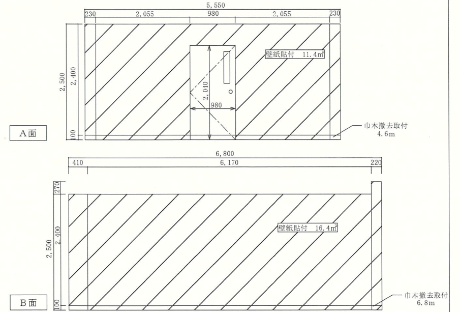
壁改修参考図 S=1/40
