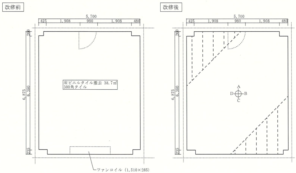
床改修参考図 S=1/60
