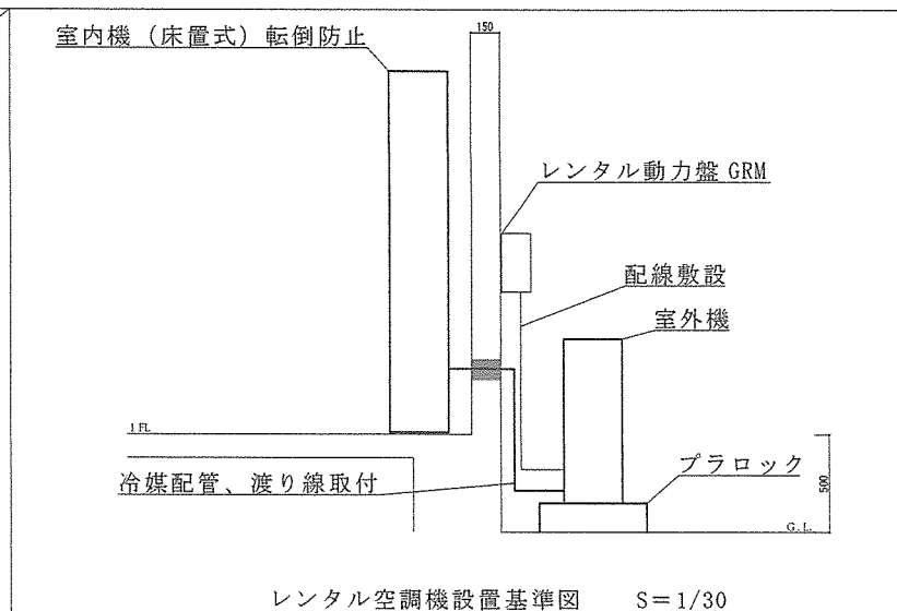
レンタル空調機設置基準図 S=1/30
