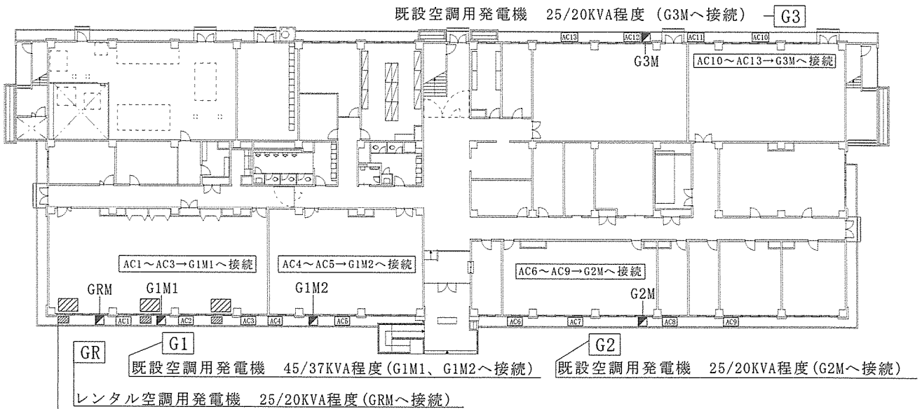
135号建物【1階】 平面図 S=1/350
