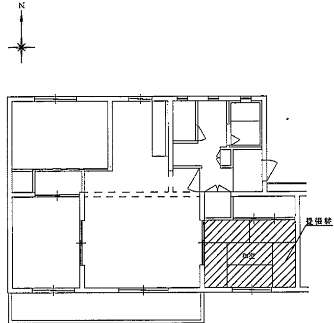
宿舍1 (生野宿舍) (D規格) 施工平面図 S=1/100
