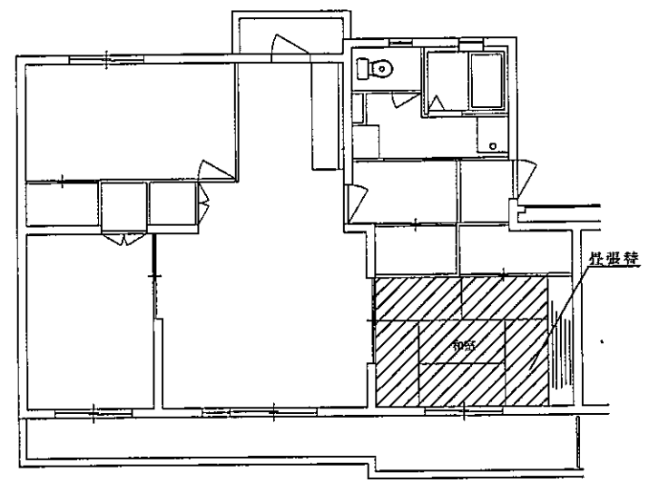
生野宿舎2棟 (D規格) 施工平面図 S=1/100
