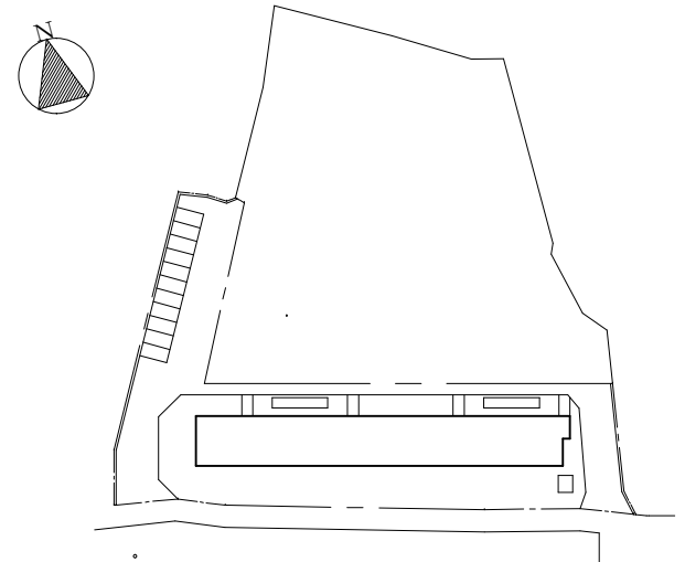
配置図 S=1:1500
