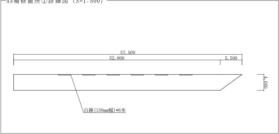
As補修箇所①詳細図 (S=1:500)
