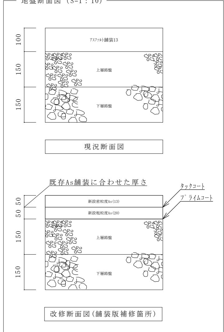
地盤断面図 (S=1:10)
