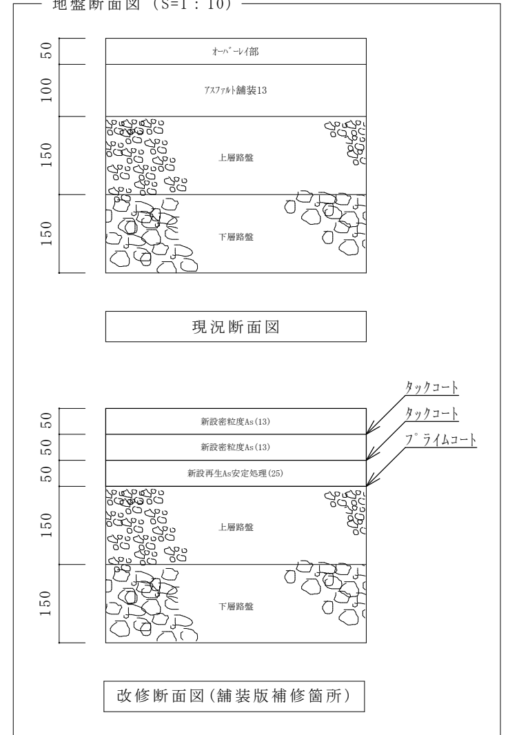
地盤断面図 (S=1:10)
