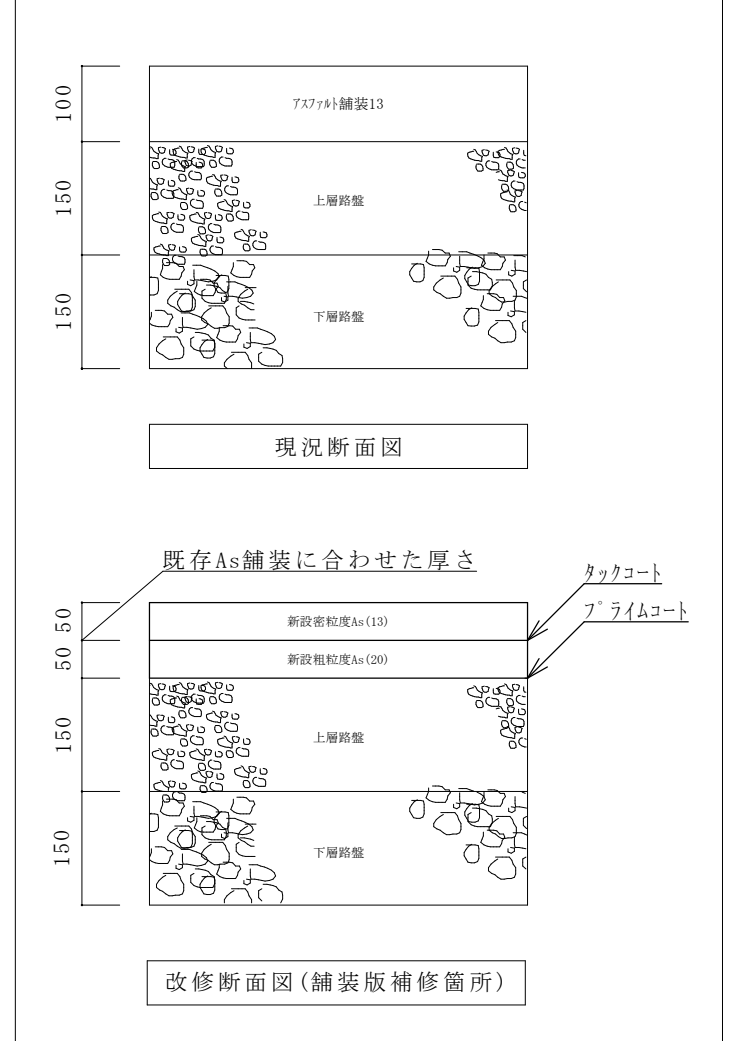
地盤断面図 (S=1:10)
