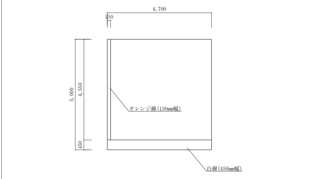
As補修箇所④詳細図 (S=1:100)
